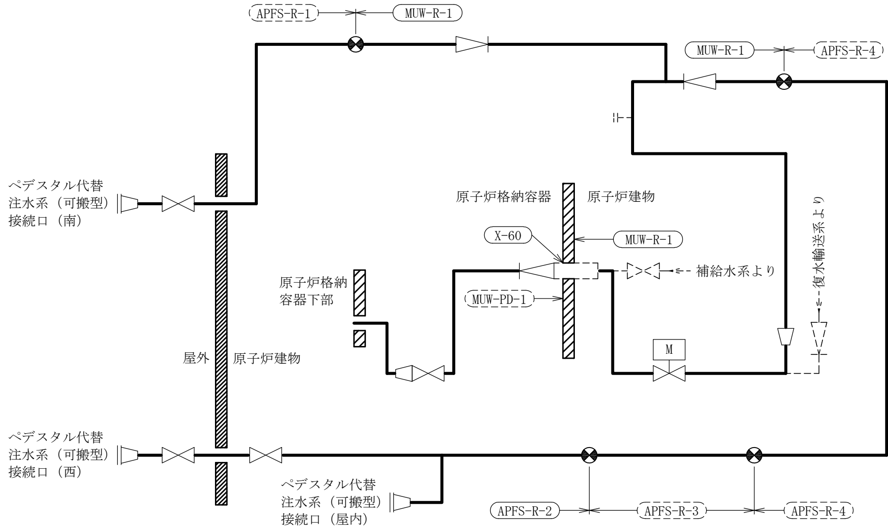
[注] 太線範囲の管クラス : SA2 ペDESTAL代替注水系概略系統図 (その1)
