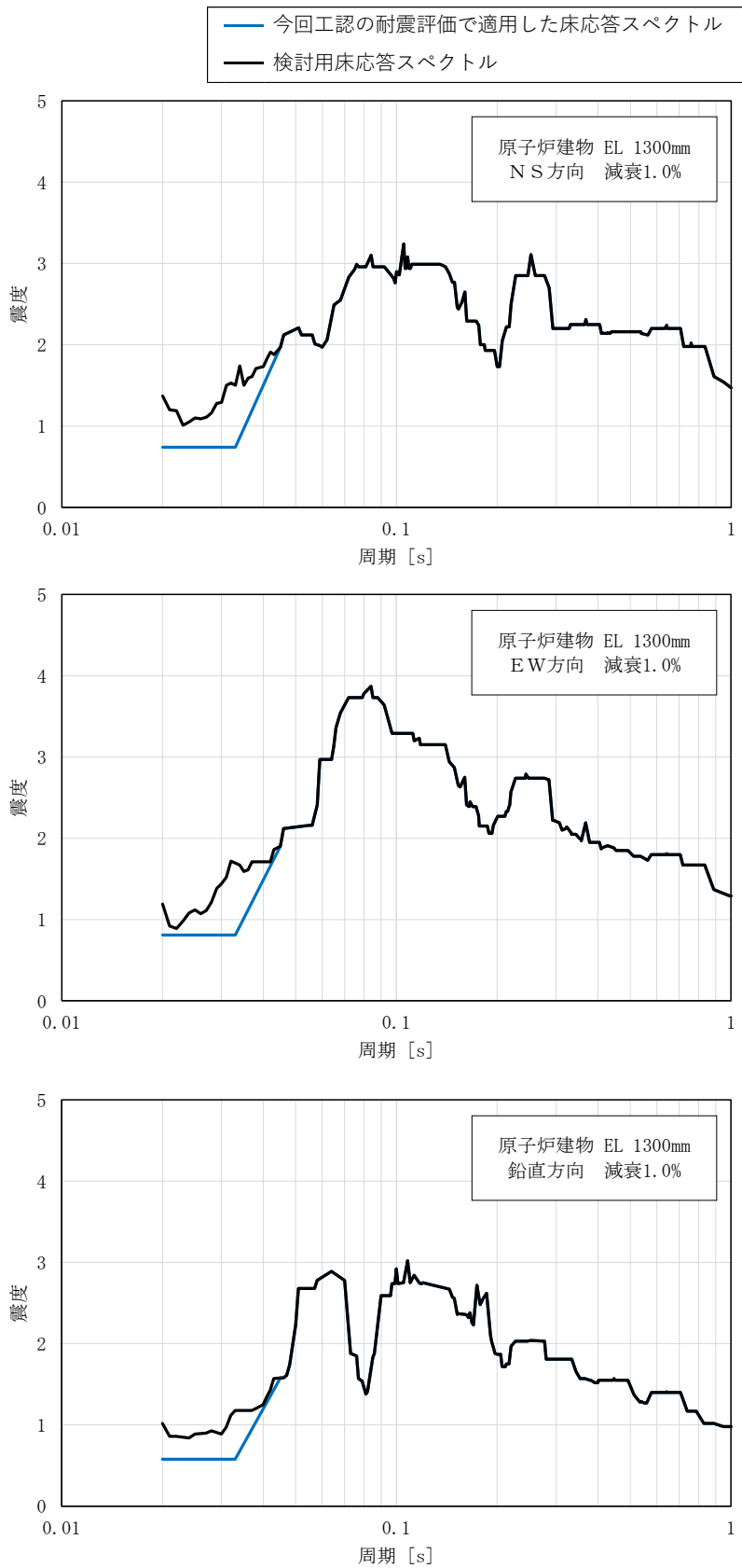
図1 検討用床応答スペクトル
