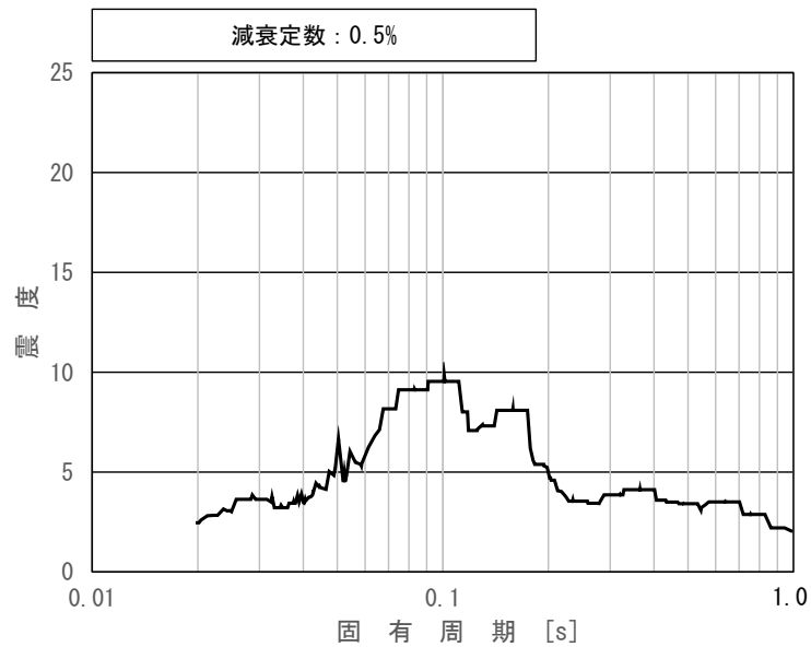
図 10 (2/2) 弁の動的機能維持評価用床応答スペクトル (基準地震動 S_s , 水平方向: 屋外配管ダクト (タービン建物~放水槽) (EW 断面) EL5.200m)
