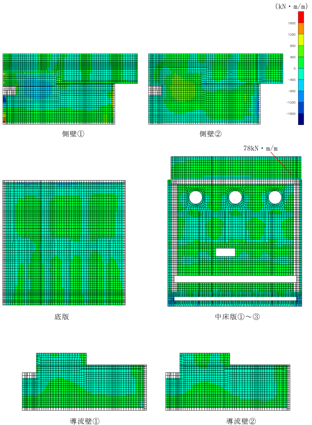
図 10-2(1) 静的地震力 (Kh=0.16 (载荷方向: 東→西)) 载荷時の断面力分布図 (曲げモーメント (kN · m/m) : My) 参考 6-17
