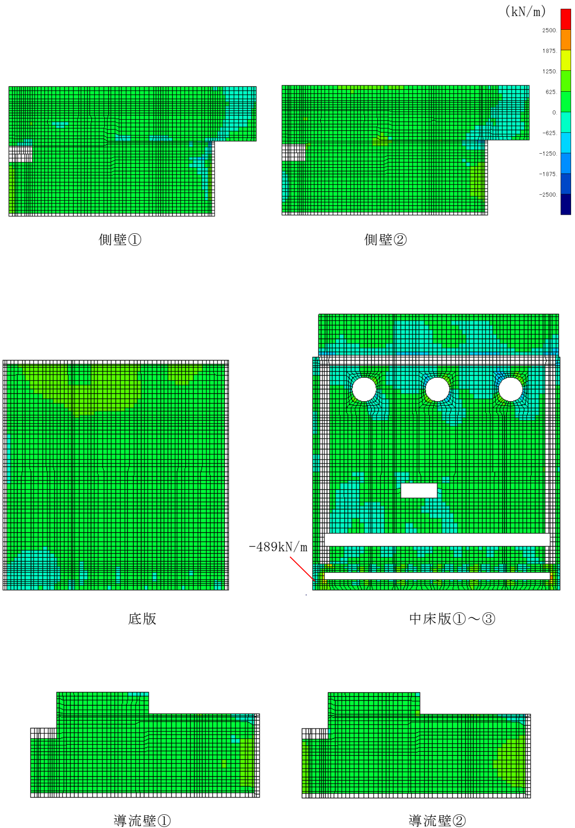
図 10-10(1) 静的地震力 ( K_h = -0.16 (荷重方向: 西→東)) 荷重時の断面力分布図 (軸力 (kN/m) : N_y , 圧縮: +) 参考 6-41
