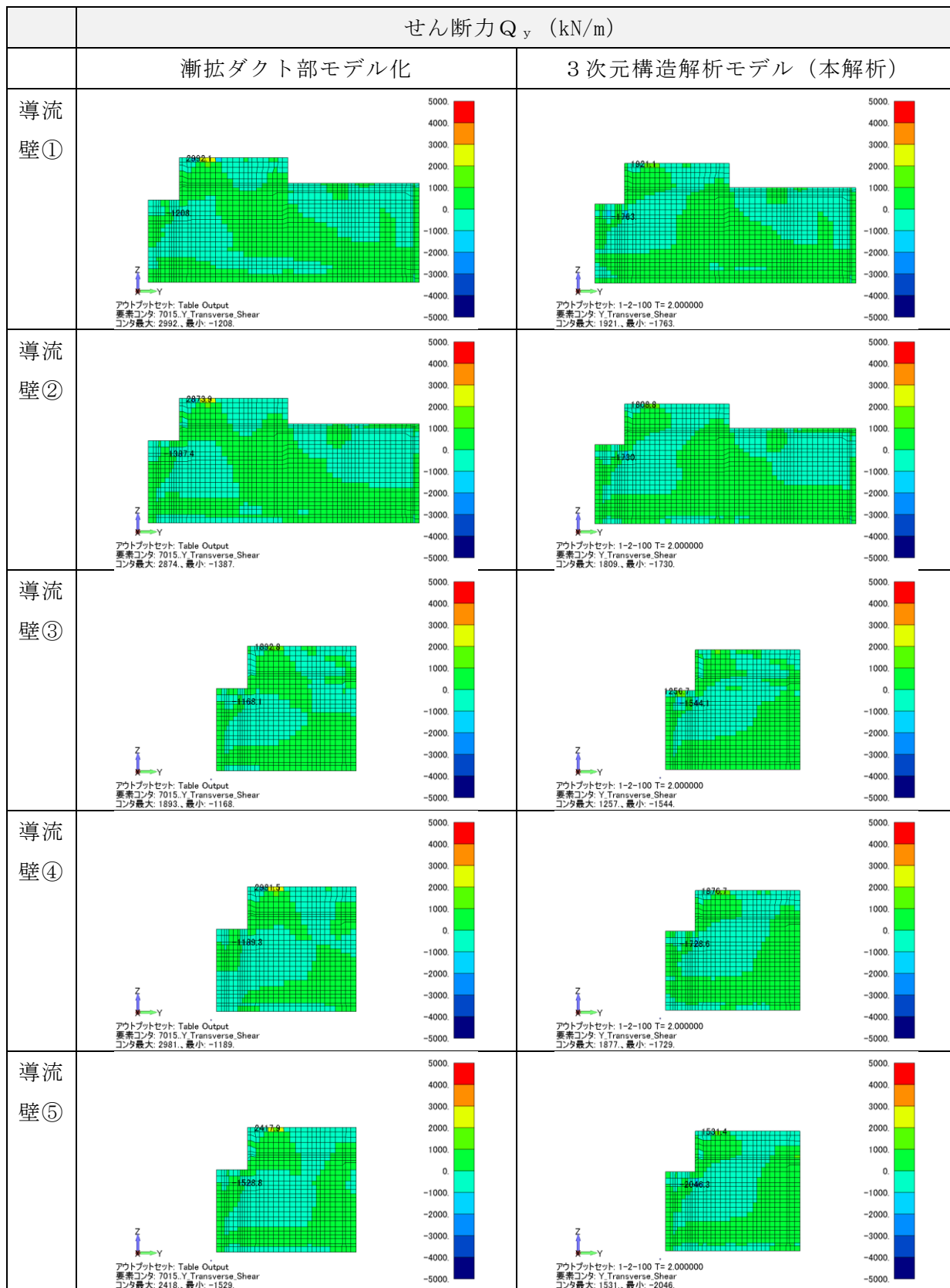
図 3-50 断面力図 (せん断力 Q_y (kN/m), No. 3)
