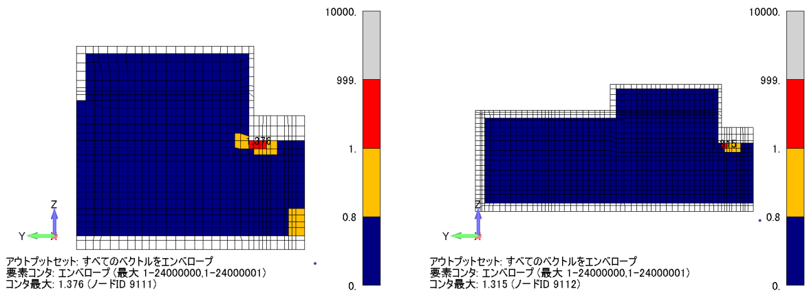
解析ケース④, S s - D (- +) 【時刻 1】
