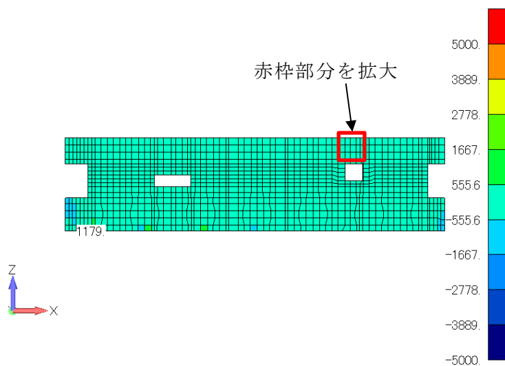
(a) せん断力分布全体図 (隔壁)
