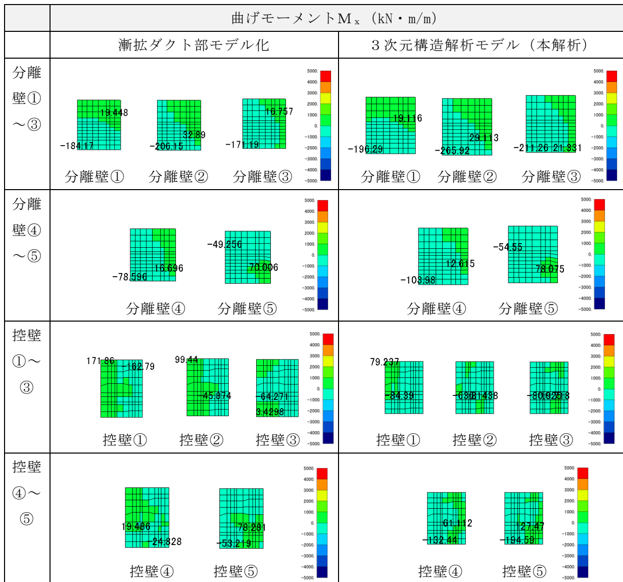
図 3-7 断面力図 (曲げモーメント M_x (kN・m/m), No. 1)
