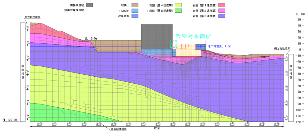
(a) 解析モデル全体図
