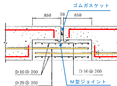
(i) 継手部付近の縦断図
