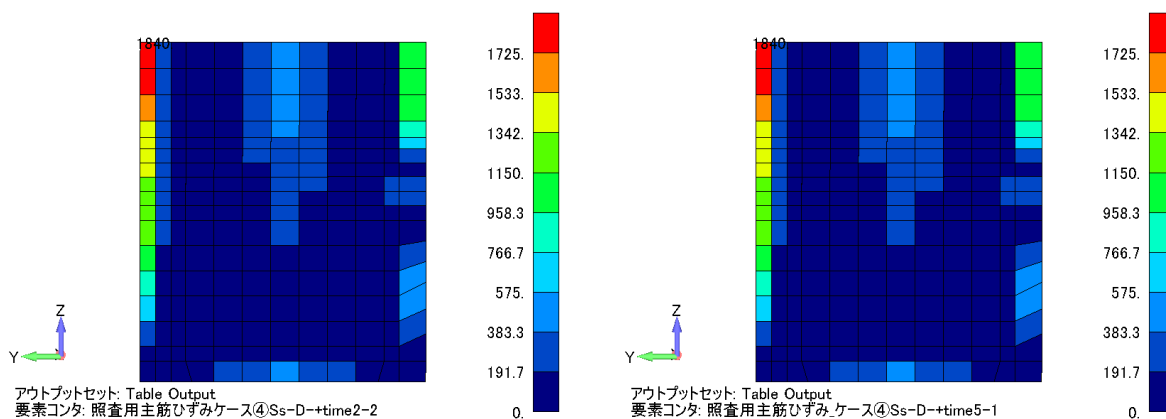
解析ケース④， S s - D（一 +） 【左：時刻 2， 右：時刻 5】
