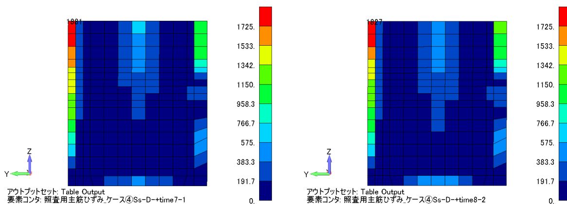
解析ケース④， S s - D（一 +） 【左：時刻 7， 右：時刻 8】
