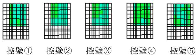
図 6-38 せん断破壊に対する照査値最大時の断面力分布図 (曲げモーメント (kN · m) : M_x ) (側壁, 解析ケース②, S_s - D (-+) )
