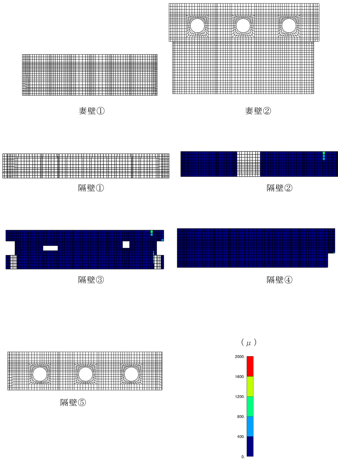
図 6-33 曲げ・軸力系の破壊に対する照査値最大時のひずみ分布図 (主筋ひずみ) (中床版, 解析ケース②, S_s - D (-+) )
