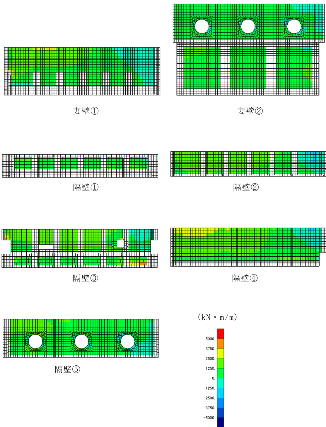
図 6-45 せん断破壊に対する照査値最大時の断面力分布図 (軸力 (kN/m) : N_x ) (側壁, 解析ケース②, S_s - D (-+))
