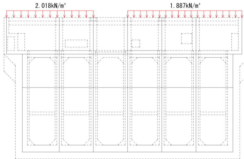
図 3-45 浸水防護施設 荷重図 (海水ポンプエリア)
