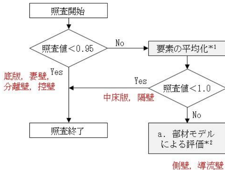
図 6-21 部材毎の最終照査方法
