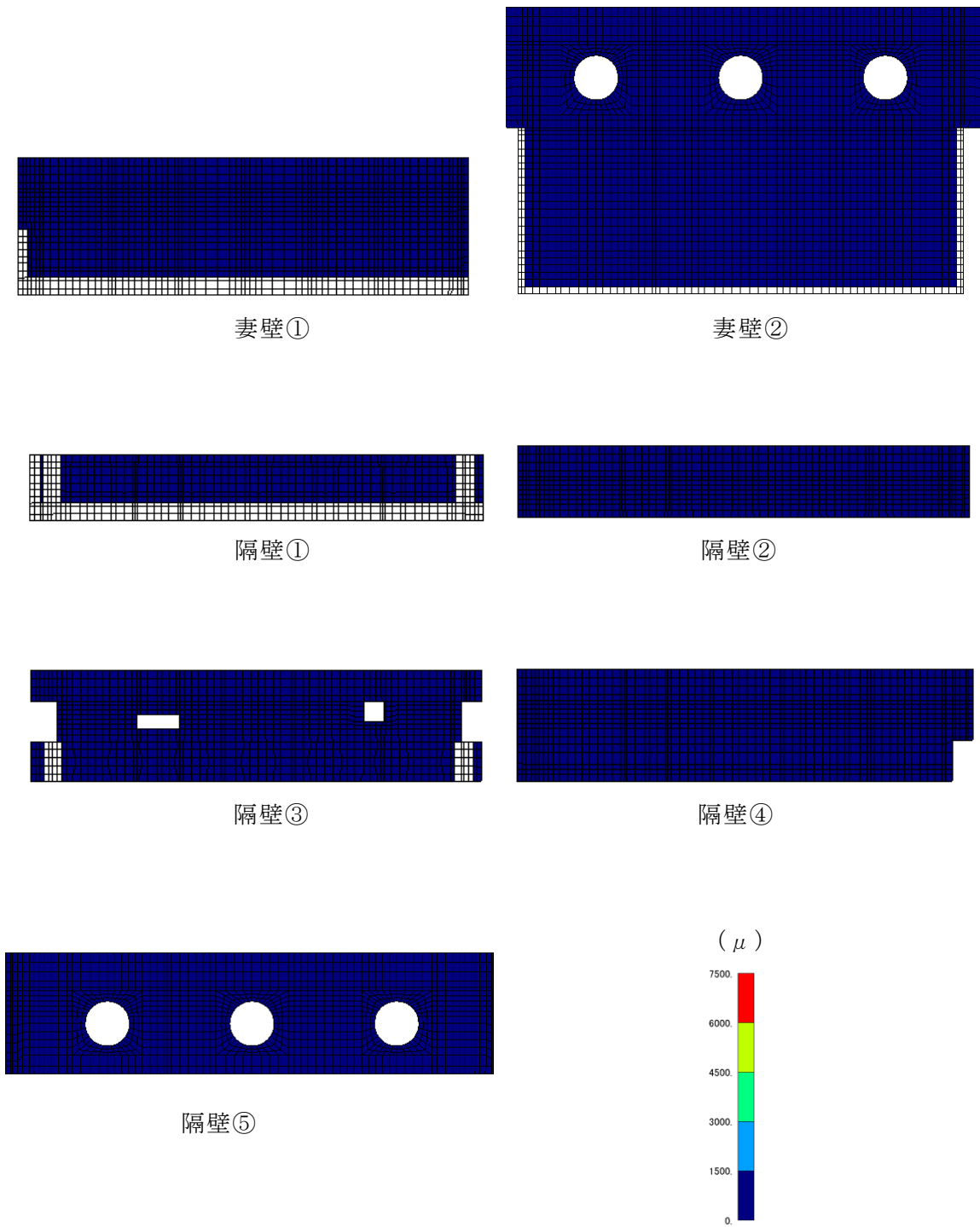
図 6-27 曲げ・軸力系の破壊に対する照査値最大時のひずみ分布図 (コンクリートの圧縮縁ひずみ) (側壁, 解析ケース④, S_s - D (-+) )
