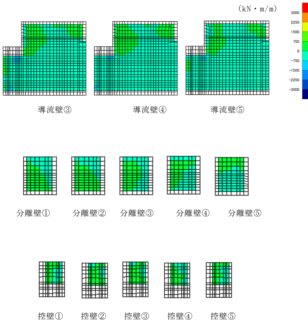
図 6-50 せん断破壊に対する照査値最大時の断面力分布図 (せん断力 (kN/m) : Q_x ) (側壁, 解析ケース②, S_s - D (-+) )
