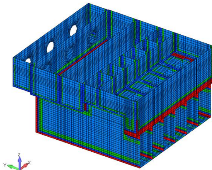
図4-5 取水槽 剛域設定範囲(赤範囲:剛域)
