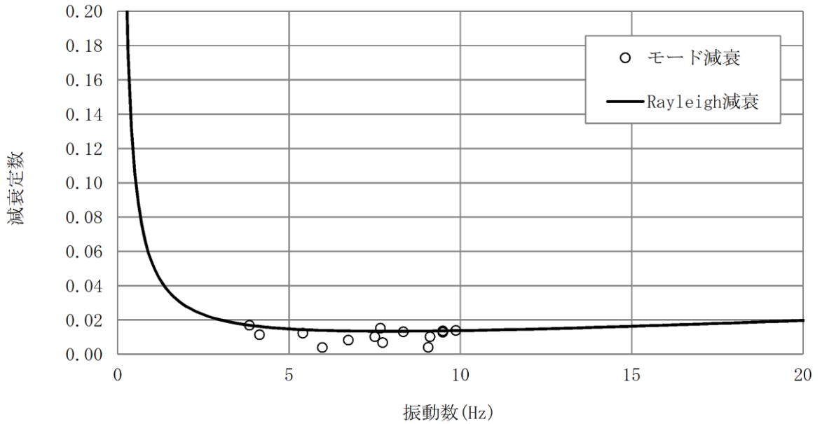
図 3-34 設定した Rayleigh 減衰 (A-A 断面)
