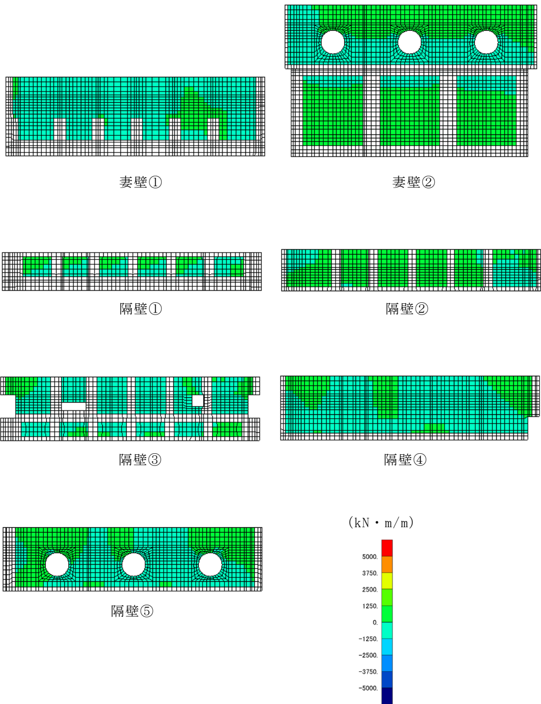
図 6-42 せん断破壊に対する照査値最大時の断面力分布図 (曲げモーメント (kN · m) : M_y ) (側壁, 解析ケース②, S_s - D (-+) )
