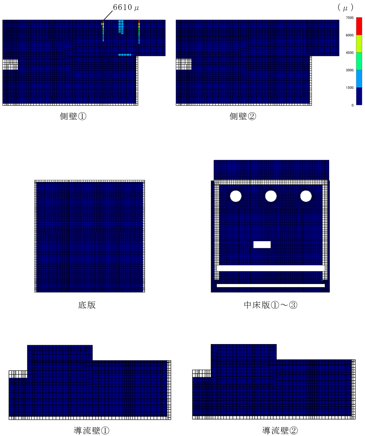
図 6-25 曲げ・軸力系の破壊に対する照査値最大時のひずみ分布図 (コンクリートの圧縮縁ひずみ) (側壁, 解析ケース④, S_s - D (-+) )
