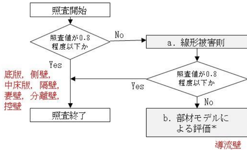
図 6-23 部材毎の最終照査方法
