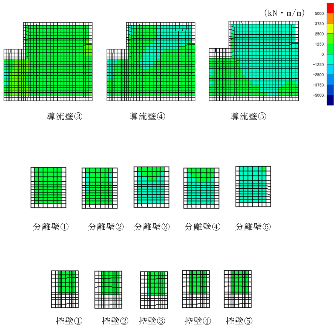
図 6-44 せん断破壊に対する照査値最大時の断面力分布図 (軸力 (kN/m) : N_x ) (側壁, 解析ケース②, S_s - D (-+) )
