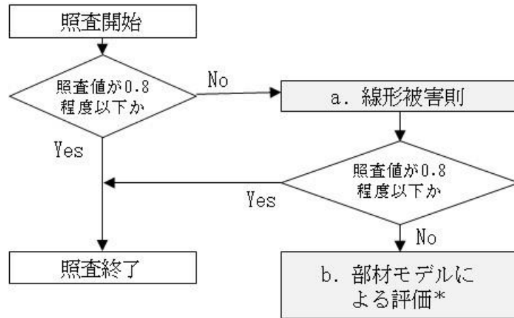
図 5-69 せん断破壊による照査フロー (PHb 設置あり) 注記* : 部材全体として終局状態に至っていないことを確認する。
