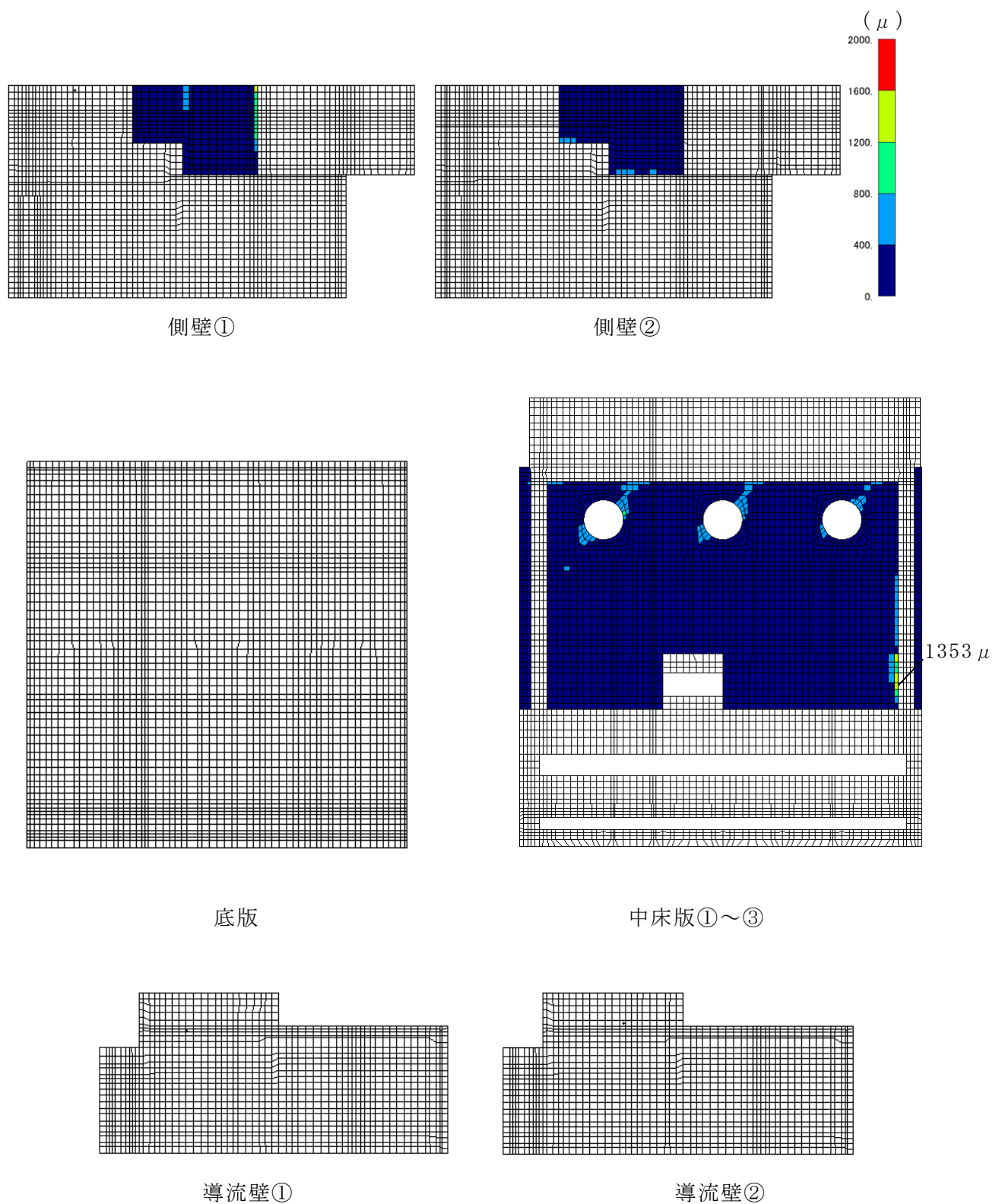
図 6-31 曲げ・軸力系の破壊に対する照査値最大時のひずみ分布図 (主筋ひずみ) (中床版, 解析ケース②, S_s - D (-+) )
