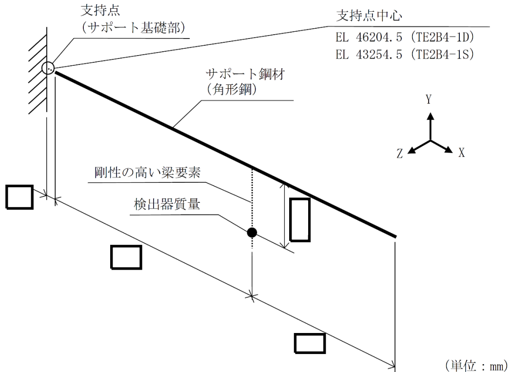
図 4-1 解析モデル
