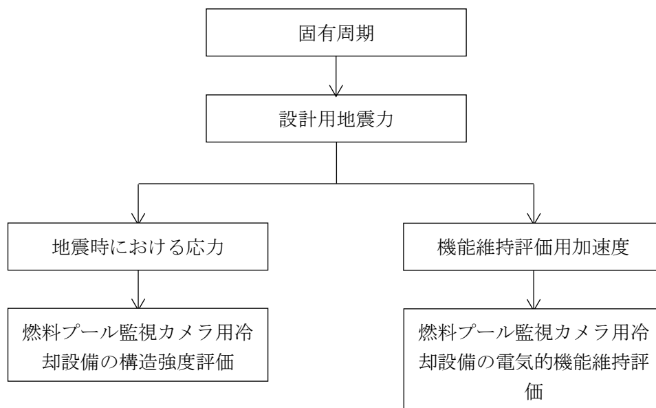
図2-1 燃料プール監視カメラ用冷却設備の耐震評価フロー
