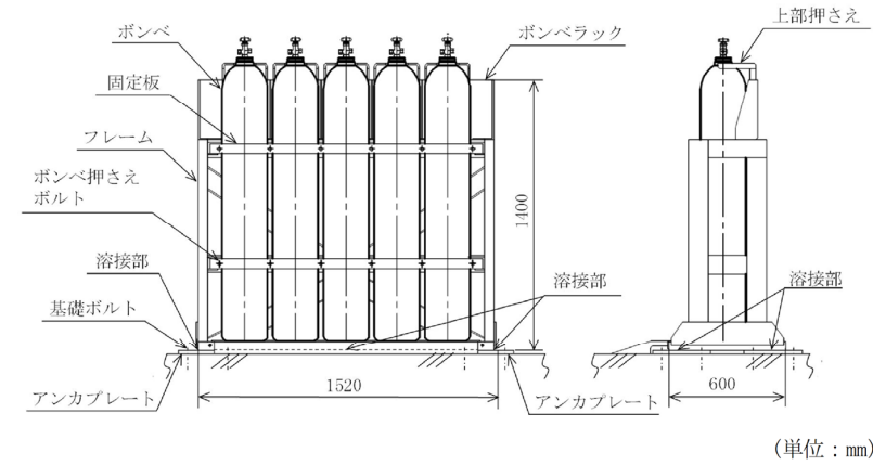
図2-2 ポンペ設備 (床固定型)
