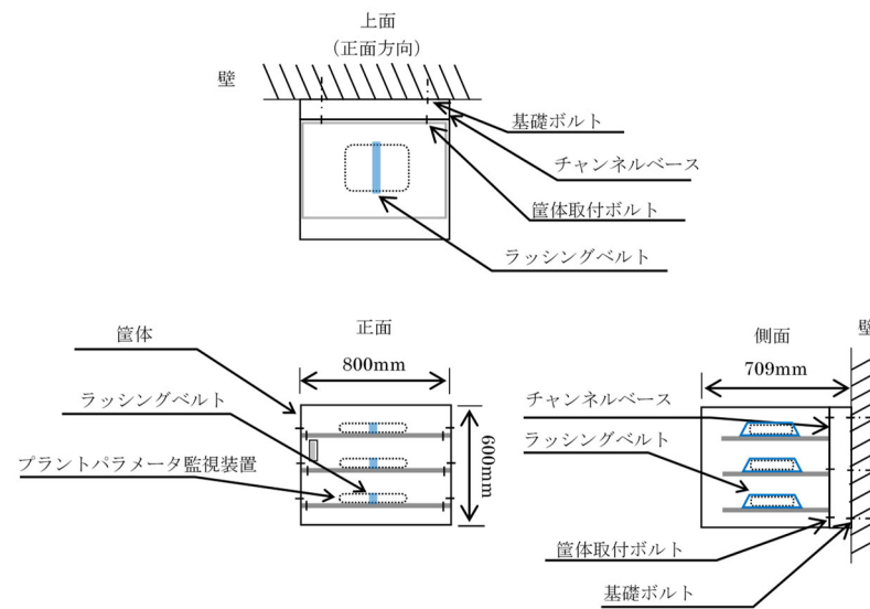
図 2-12 その他設備 (筐体固縛保管)
