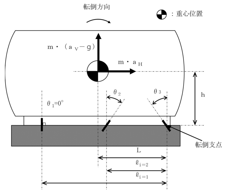
図 4-10 直接支持構造物の計算モデル例(2/2)
