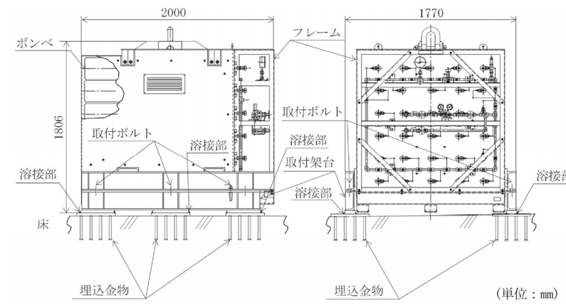
図2-4 ポンベ設備 (ポンベカードル)
