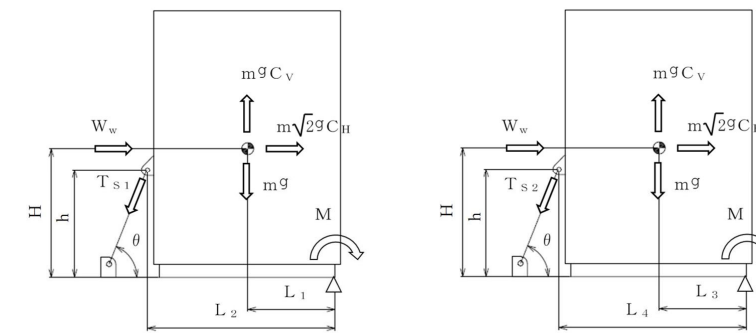
図 4-24 計算モデル (緊急時対策所空気浄化フィルタユニットの機器固縛金具)
