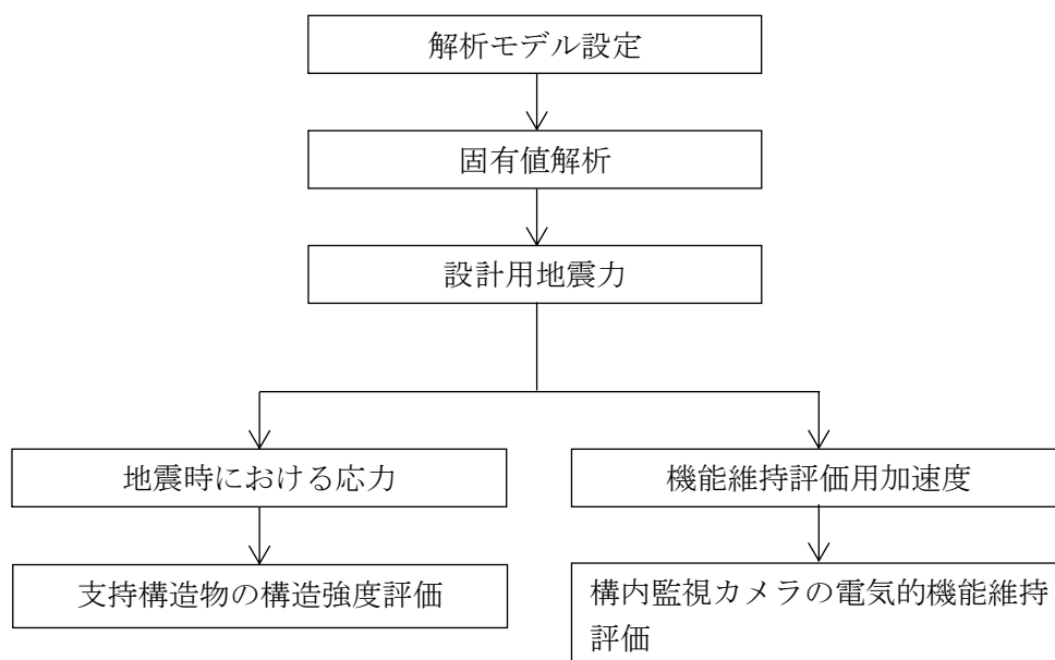
図 2-1 構内監視カメラの耐震評価フロー
