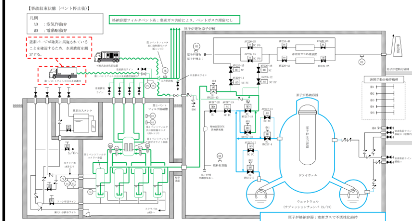
図1-12 水素爆発防止対策 (事故収束状態 (ベント停止後))
