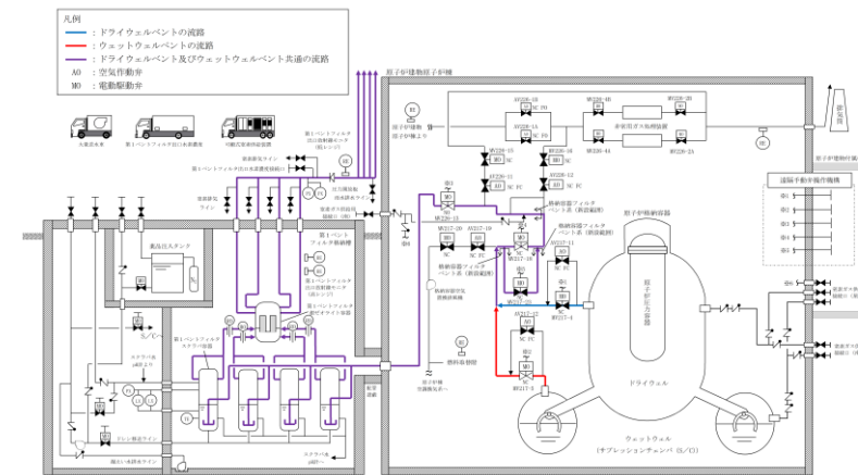
図1-1 格納容器フィルタベント系 系統概要図
