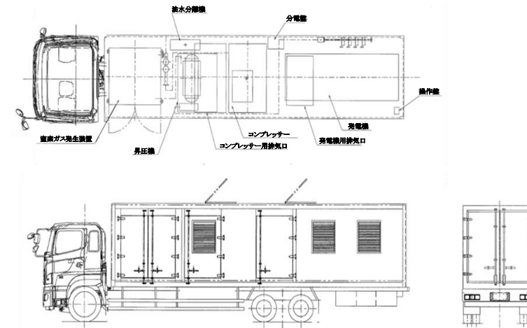
図2-41 可搬式窒素供給装置構造図
