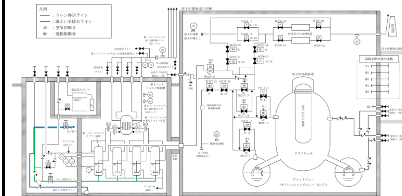
図2-43 排水設備概要図
