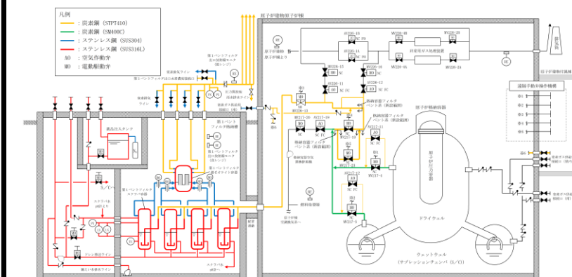
図2-2 第1ペントフィルタスクラバ容器、第1ペントフィルタ銀ゼオライト容器及び配管の材料範囲
