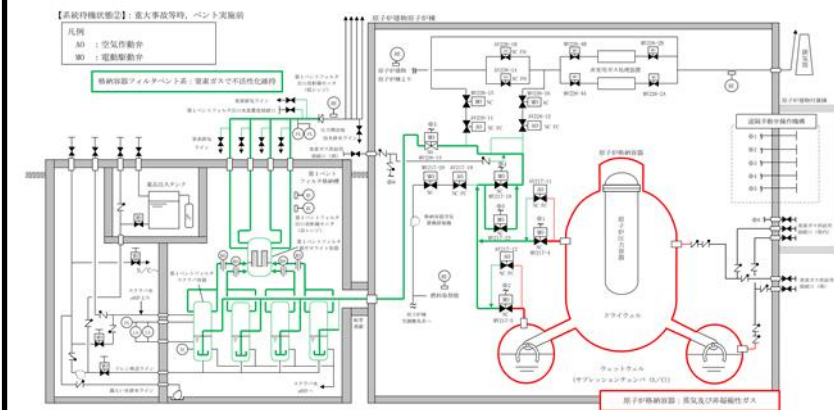
図1-2 水素爆発防止対策 (系統待機状態②)
