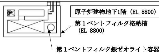
図 2-14 第1 ベントフィルタスクラバ容器及び第1 ベントフィルタ銀ゼオライト容 器の配置図
