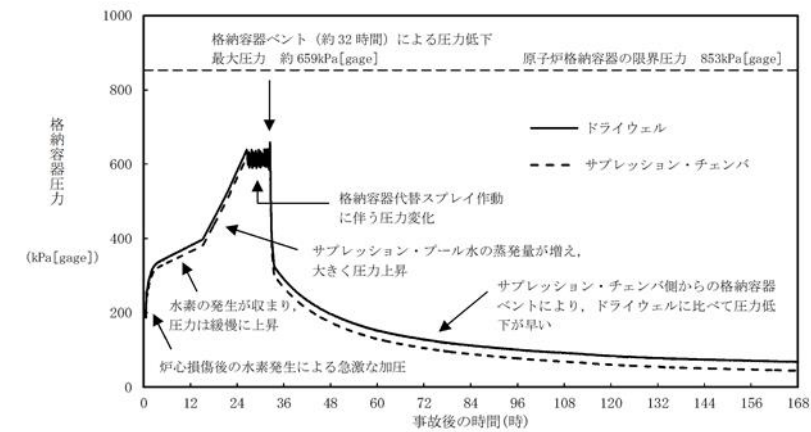
図2-2 「冷却材喪失(大破断LOCA)+ECCS注水機能喪失+全交流動力電源喪失」時における格納容器圧力の推移
