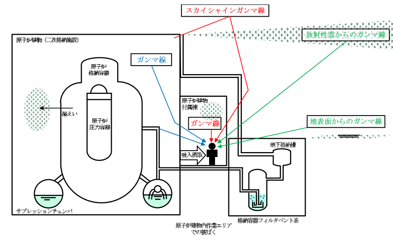
図 5-1 被ばく経路概念図 (屋内)
