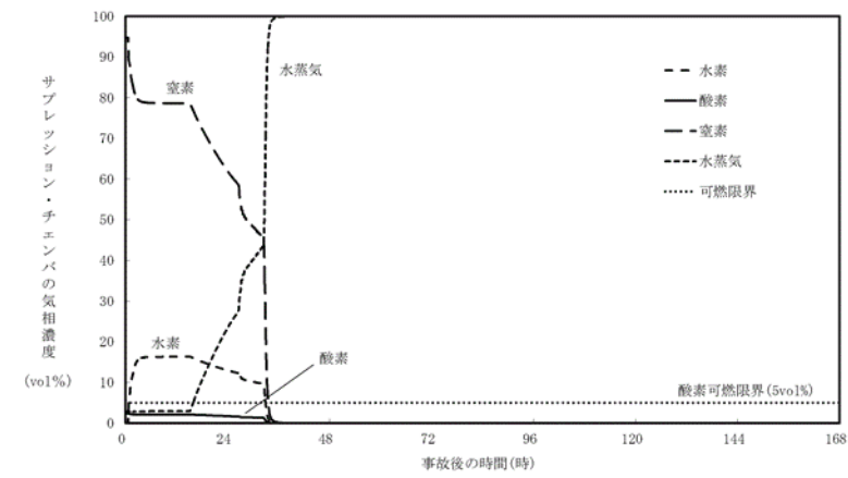
図1-9 格納容器過圧・過温破損モード (冷却材喪失 (大破断LOCA) + ECCS注水機能喪失 + 全交流動力電源喪失) におけるサブプレッションチェンバの気相濃度の推移 (ウェット条件)
