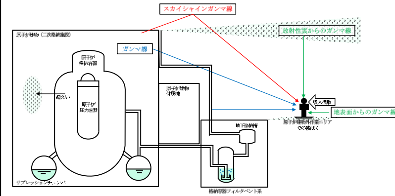
図 5-2 被ばく経路概念図 (屋外)
