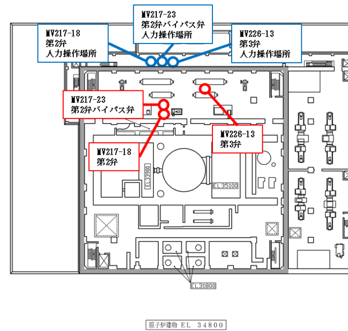
図1-4 隔離弁の操作場所 (原子炉建物3階)
