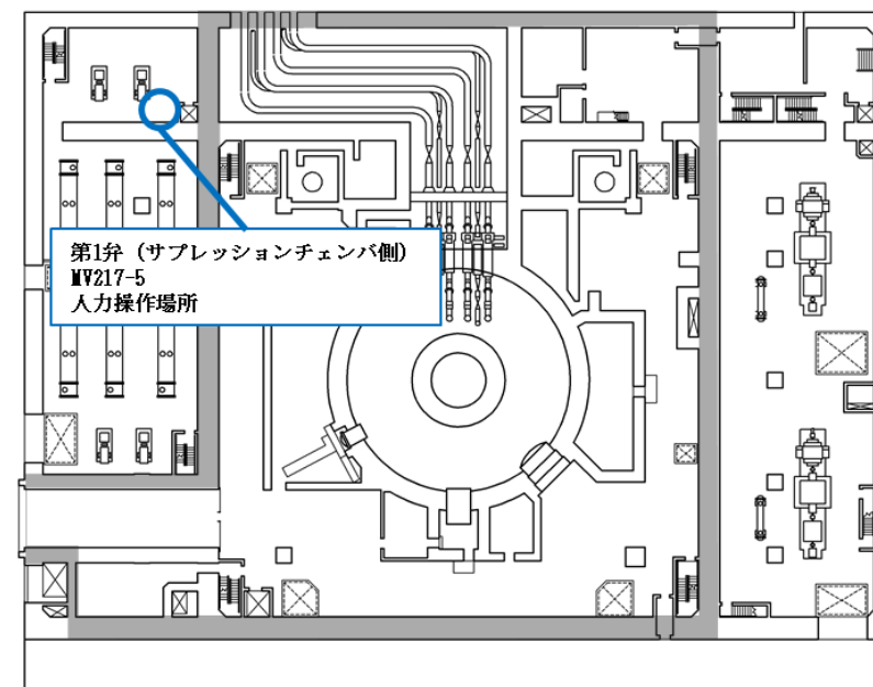
原子炉建物 EL 15300
