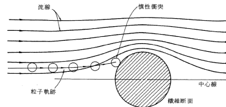
図3-3 慣性衝突による捕集
