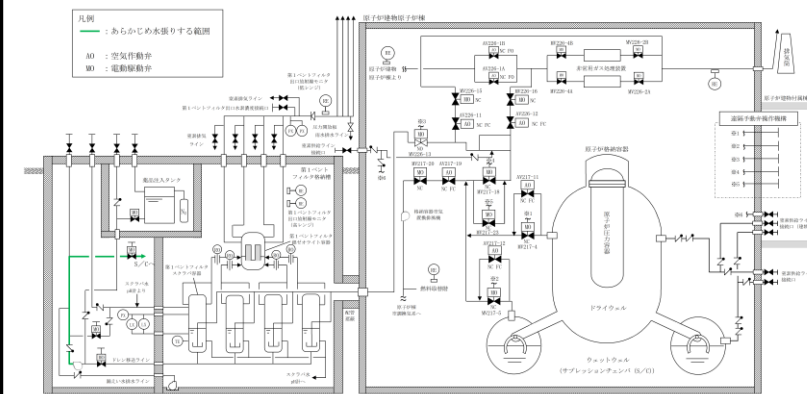
図1-10 ドレン移送ライン水張り範囲系統図
