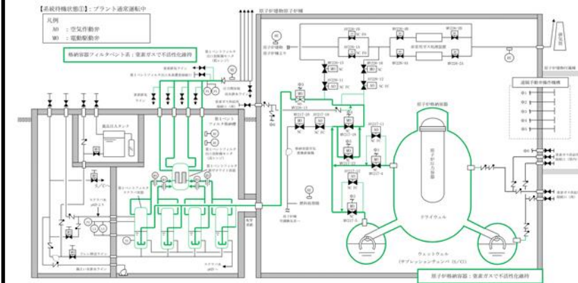
図1-1 水素爆発防止対策 (系統待機状態①)
