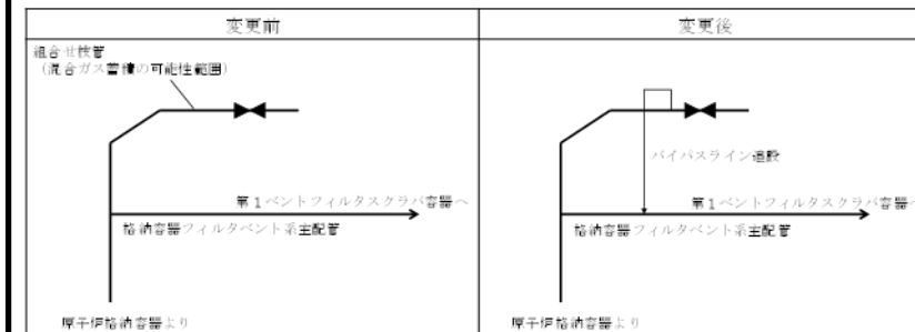
図1-4 枝管へのバイパスラインの追設 (混合ガス蓄積防止)
