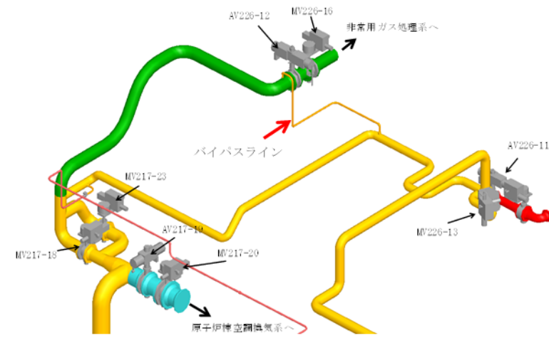
図1-5 追設するバイパスラインの鳥瞰図
