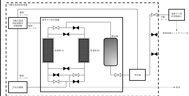
図2-42 可搬式窒素供給装置構成概略図
