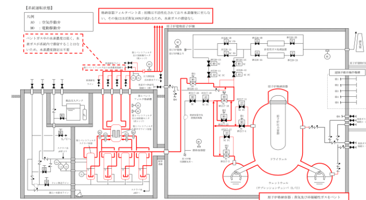
図1-6 水素爆発防止対策(系統運転状態)
