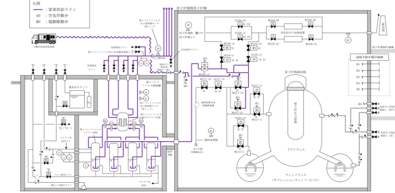
図2-40 可搬式窒素供給装置概要図
