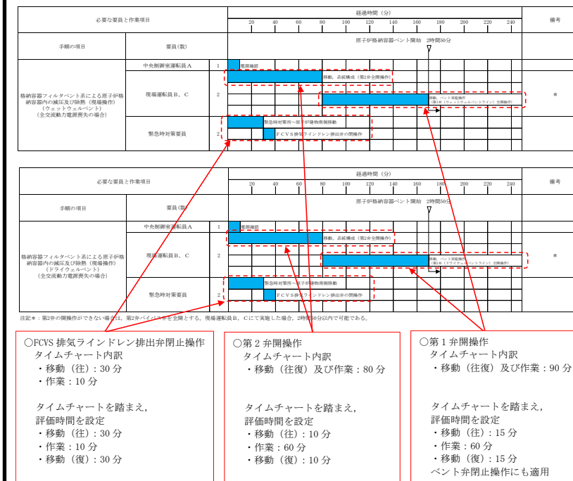
図 1-6 ベント実施に伴う現場作業のタイムチャート (1/2)
