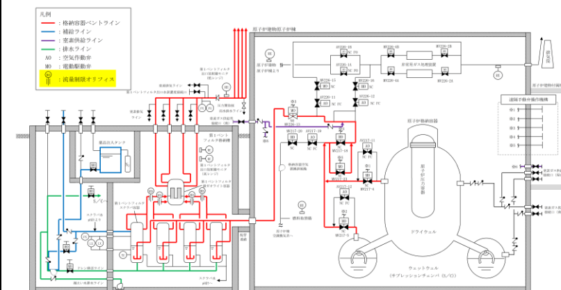
図2-1 格納容器フィルタベント系 系統概要図
