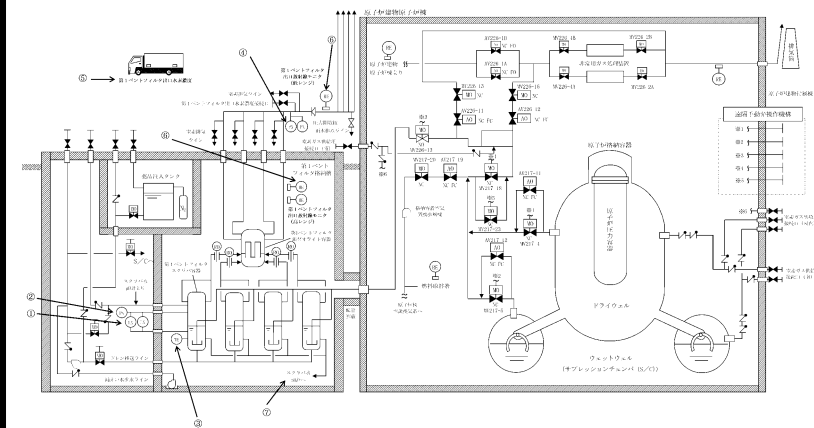
図2-36 格納容器フィルタベント系の計装設備 概略構成図
