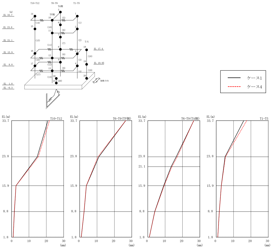
図 2-56 最大応答変位 (基準地震動 S s - D, N S 方向)
