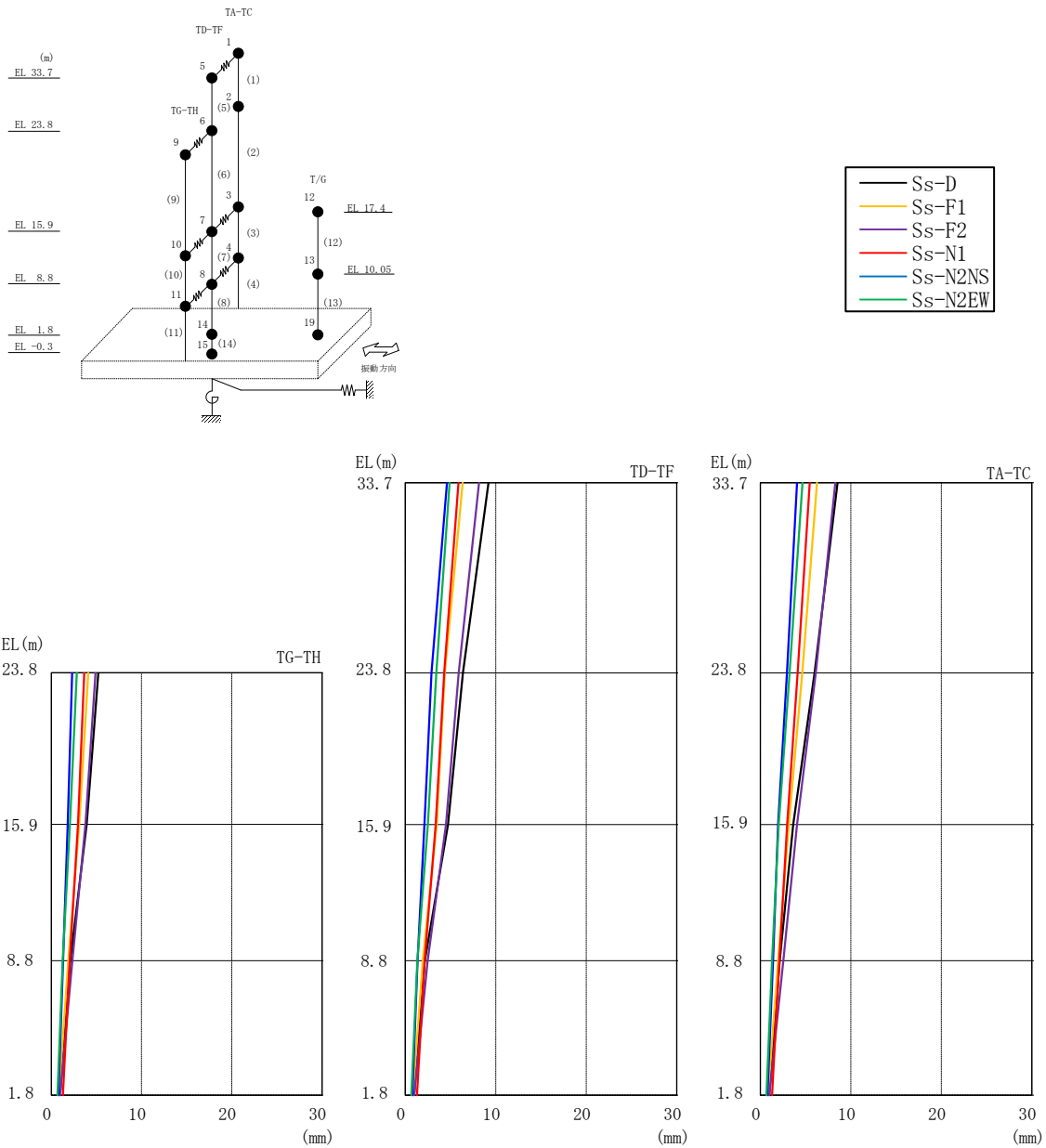
図 3-6 最大応答変位 (基準地震動 S_s , EW方向)
