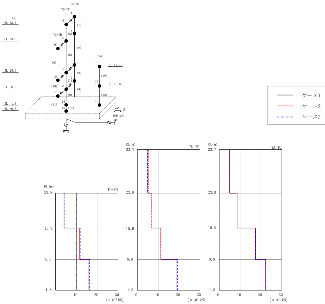
図 2-33 最大応答せん断力 (基準地震動 S s -F 2, EW 方向)
