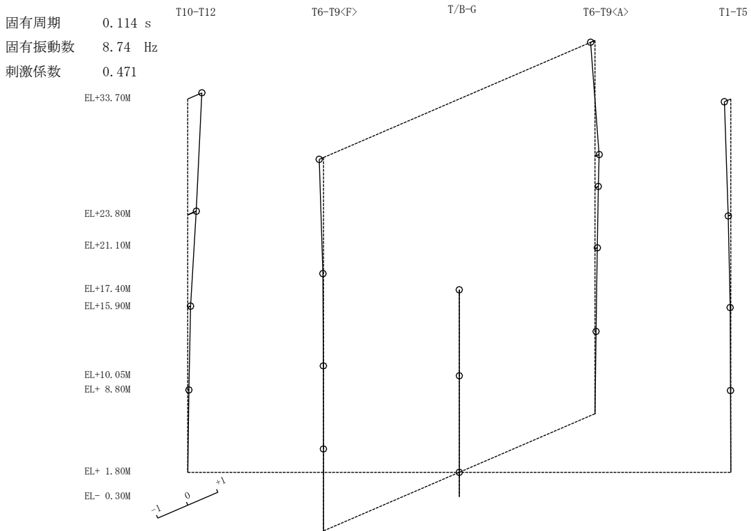
4次 モード
