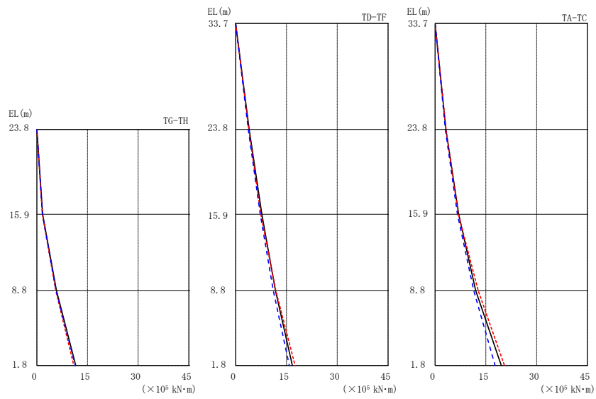
図 2-40 最大応答曲げモーメント (基準地震動 S_s - N2NS , EW方向)
