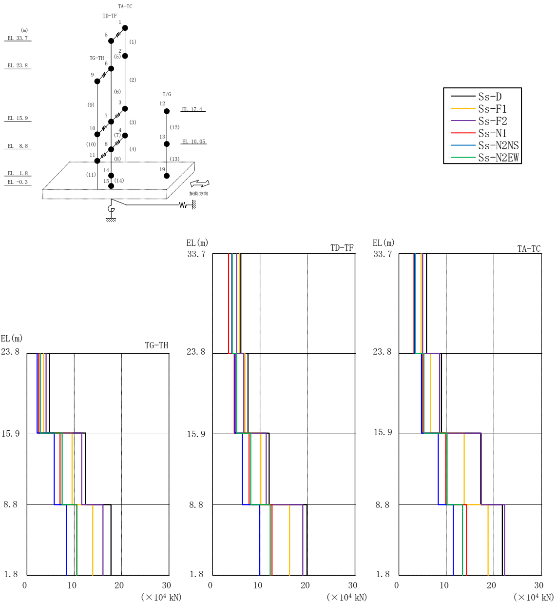
図 3-7 最大応答せん断力 (基準地震動 S_s , EW 方向)
