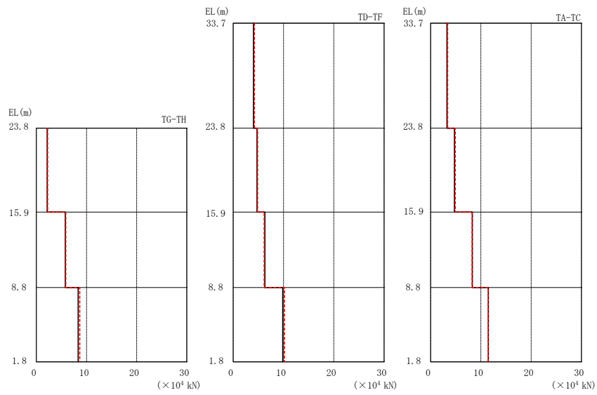
図 2-85 最大応答せん断力 (基準地震動 S_s - N2NS , EW方向)
