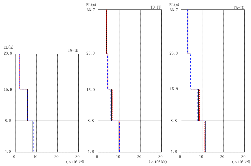
図 2-35 最大応答せん断力 (基準地震動 S s -N2NS, EW方向)
