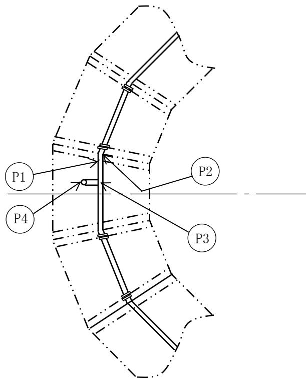
図 4-2 サプレッションチェンバスプレイ管の応力評価点
