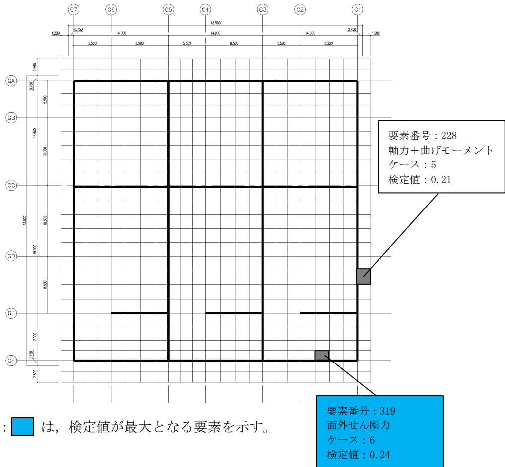
図 2-2 断面力ごとの検定値が最大となる要素及び断面の評価結果
