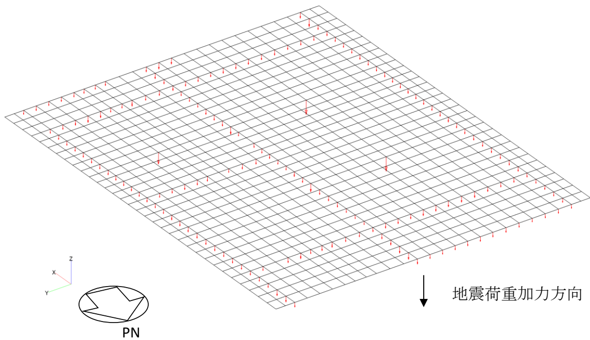
(e) 鉛直力
