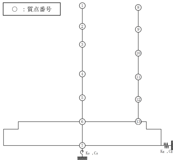
参考図1 3号復水貯蔵タンクの地震応答解析モデル （3号復水貯蔵タンク基礎のモデル図（水平方向））
