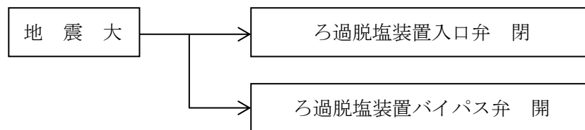
図 4-18 燃料プール冷却系弁閉止システムの弁動作インターロック
