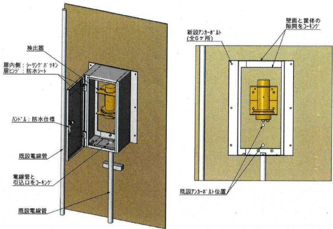
図 4-22 被水防護カバーの概要図
