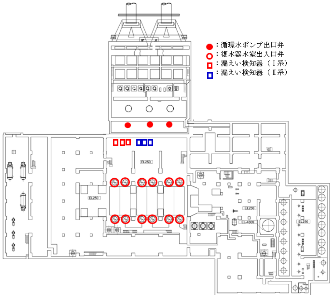
図 4-19 漏えい検知器，循環水ポンプ出口弁及び復水器水室出入口弁の配置図
