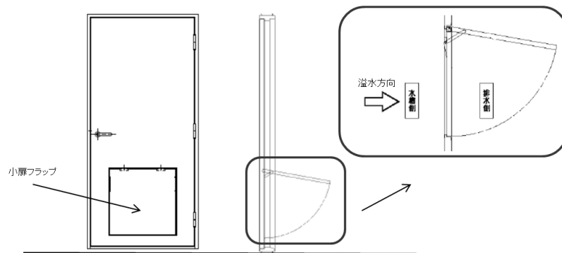
図4-24 通水扉の概要図
