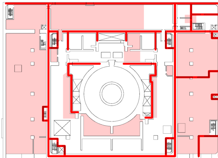
原子炉建物 EL. 23800
