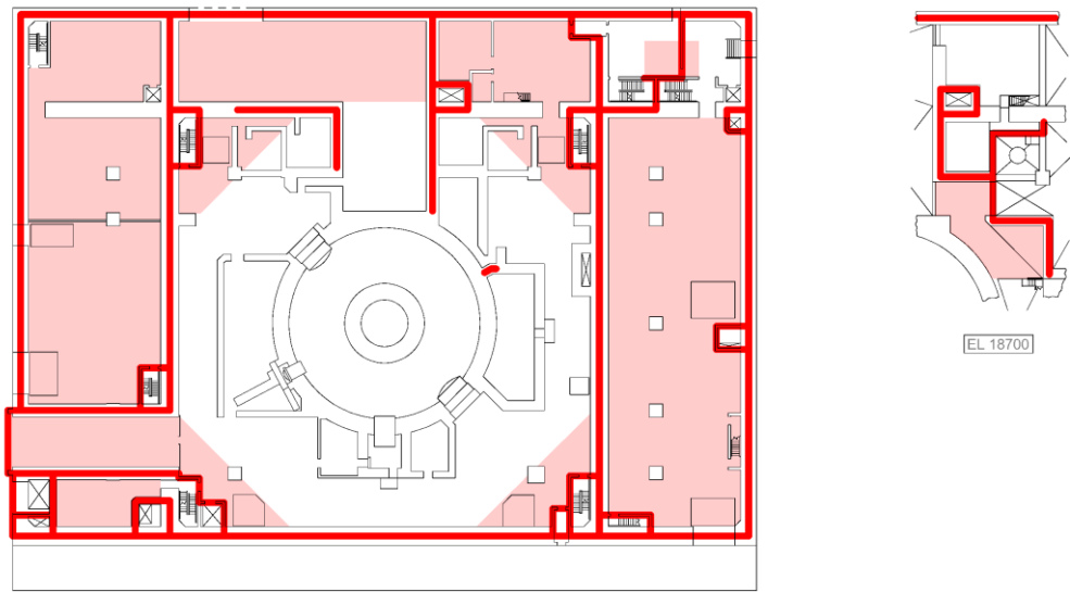
原子炉建物 EL. 15300
