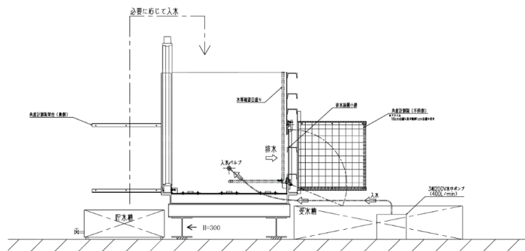
図 4-27 通水試験概要図
