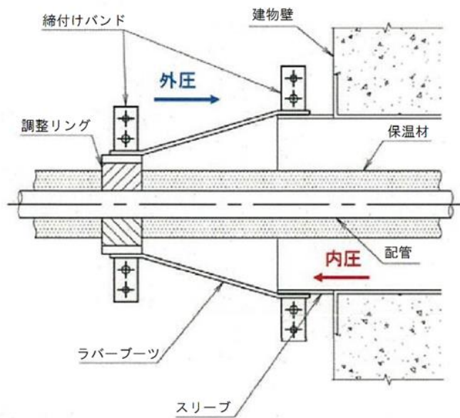
図 4-11 漏えい試験概要図 (ブーツ)
