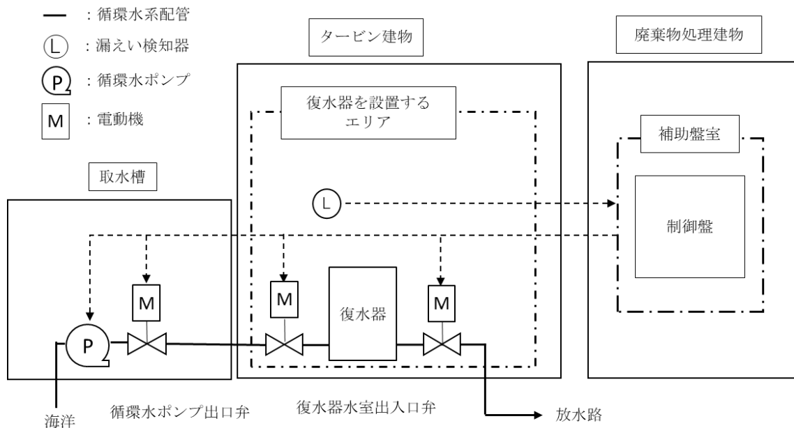
図 4-20 循環水系隔離システムの概要
