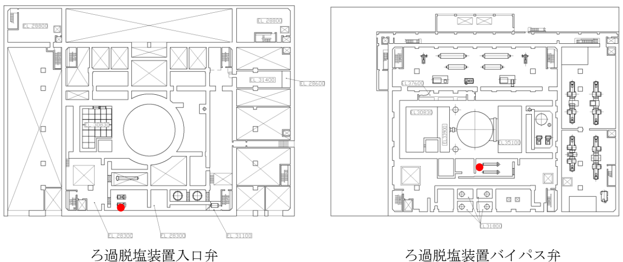
図4-16 燃料プール冷却系弁閉止システムの遮断弁配置図
