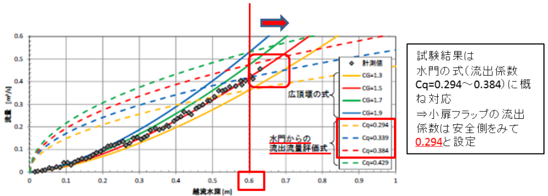
図4-30 流出係数の設定(水門の式)
