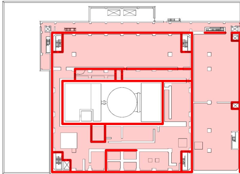
原子炉建物 EL 30500
