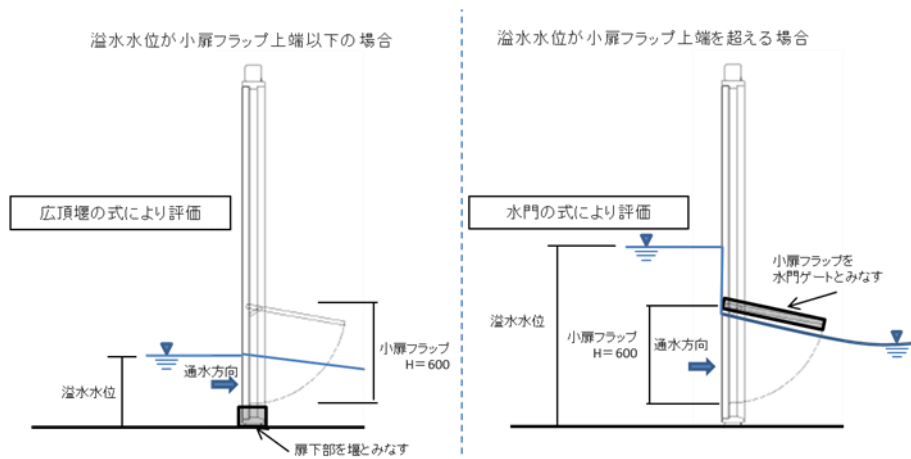
図 4-26 排水量評価式の適用状況
