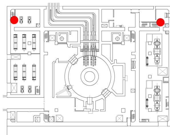
原子炉建物 EL 15300
