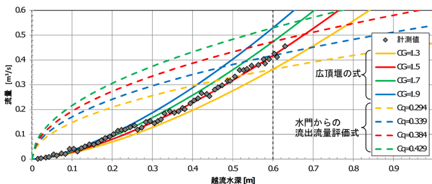
図 4-28 通水扉越流水深と流量の関係
