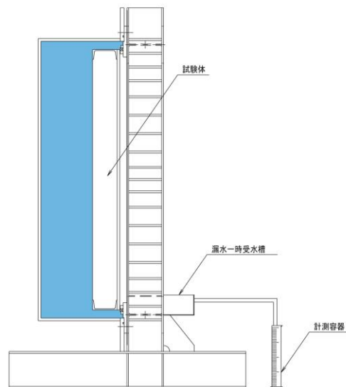
図 4-1 溢水用水密扉の漏えい試験概要図
