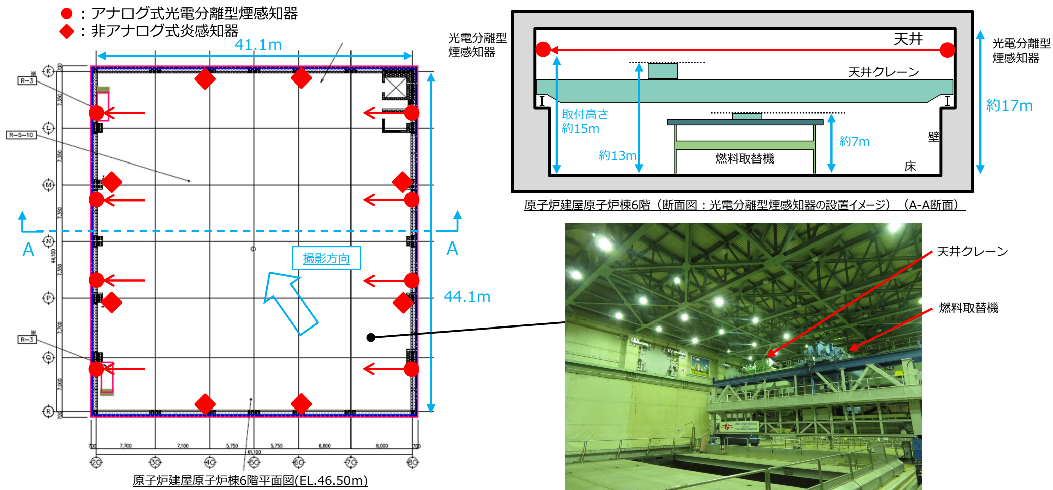
図4 原子炉建屋原子炉棟6階（オペレーティングフロア）
