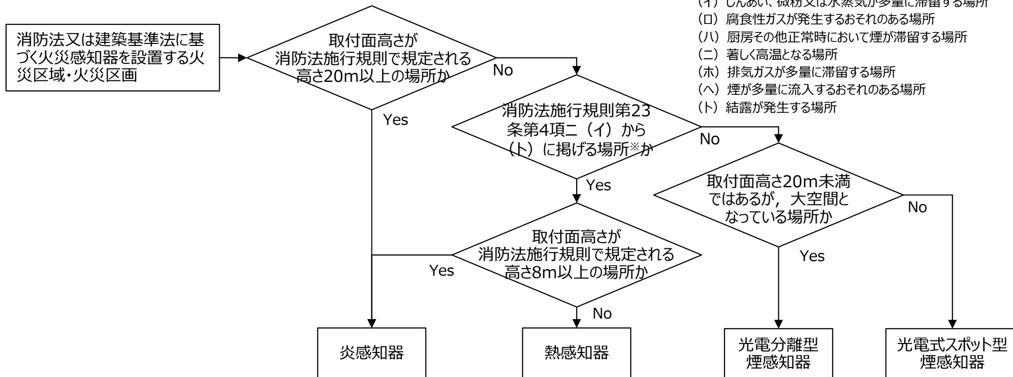
図7 消防法又は建築基準法に基づき火災感知器を1種類設置する火災区域・火災区画の火災感知器の選択フロー
