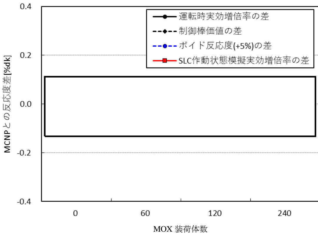
図 3-32 全炉心 MCNP 妥当性確認結果 (MCNP との反応度差[%Δk])
