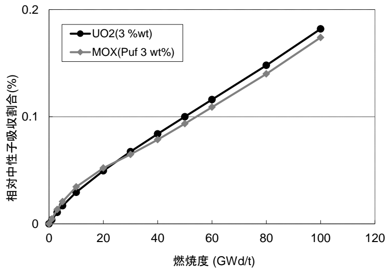
図 3.1-12 全中性子吸収に占める擬似 FP 核種の相対吸収割合
