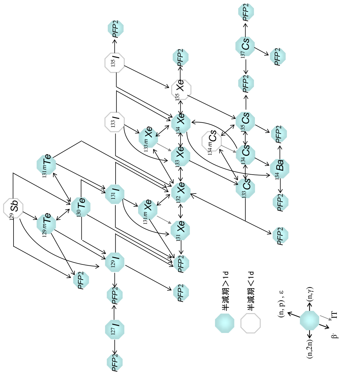
図 3.1-15 核分裂生成核種の生成・崩壊チェーン (その 2)
