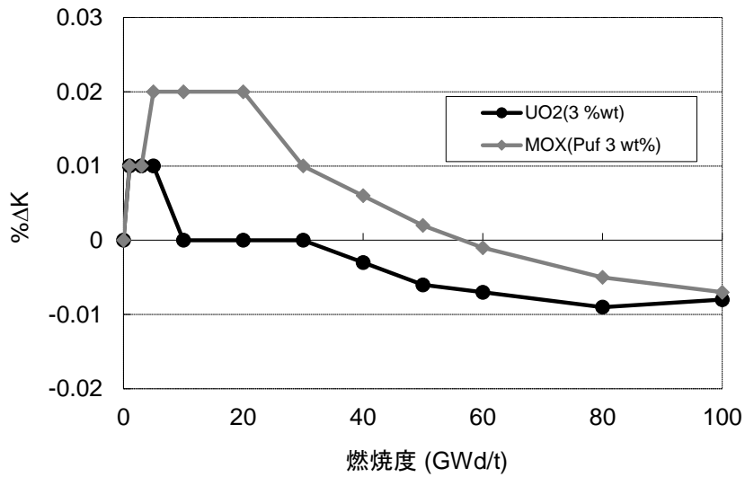
図 3.1-11 FP チェーンモデルの不確かさ
