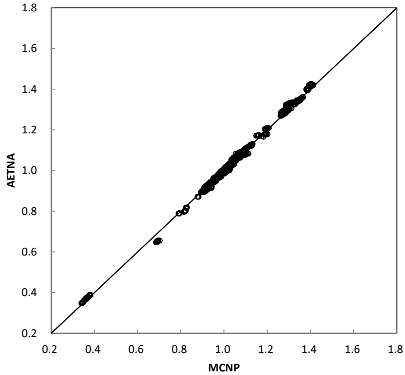
図 3-20 10×10 燃料平衡炉心問題の全燃料棒の局所出力分布の比較 (炉心 1)
