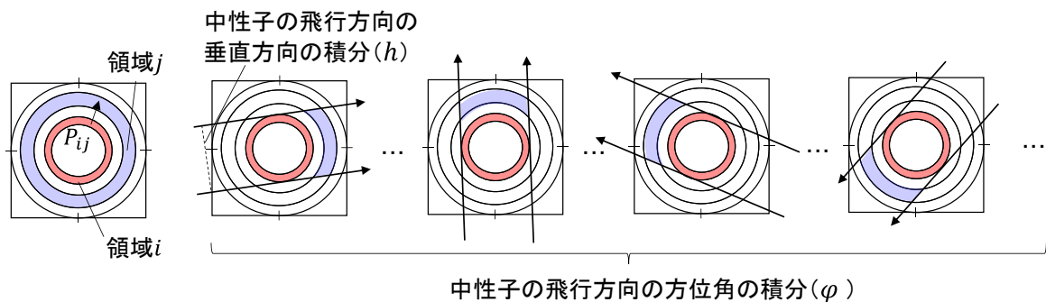
図 3.1-7 衝突確率の数値積分
