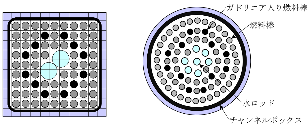
図 3.1-1 燃料集合体実形状と円筒クラスタ体系（9 × 9 燃料の例）
