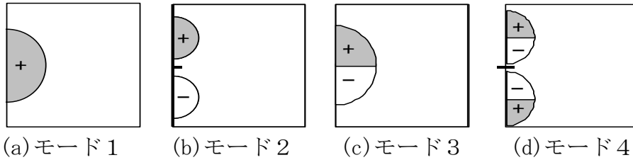
図 3.1-10 流入中性子流のモード
