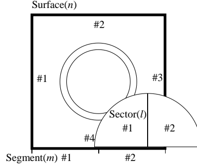
図 3.1-8 ノード表面及び角度領域の分割
