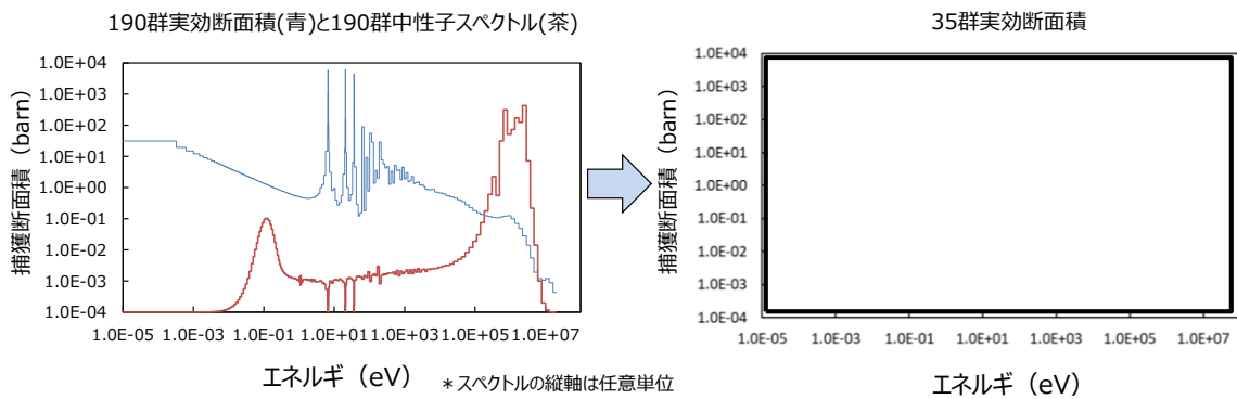
図 1.4-4 中間エネルギー群（35 群）実効断面積の計算の概要
