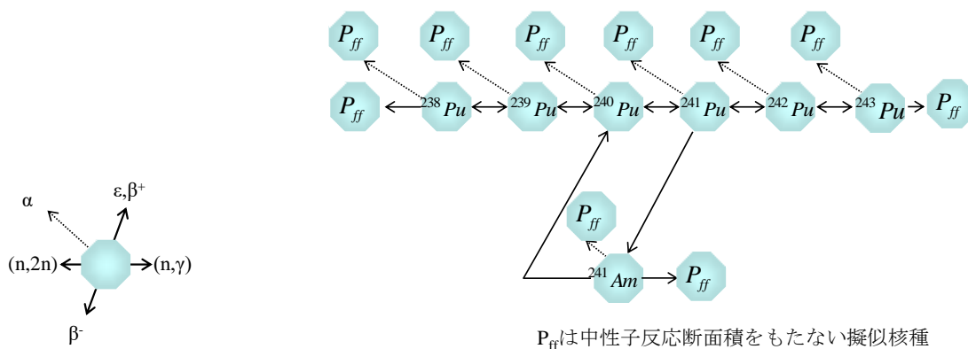
図 3.1-18 プルトニウム起源対象核種チェーン
