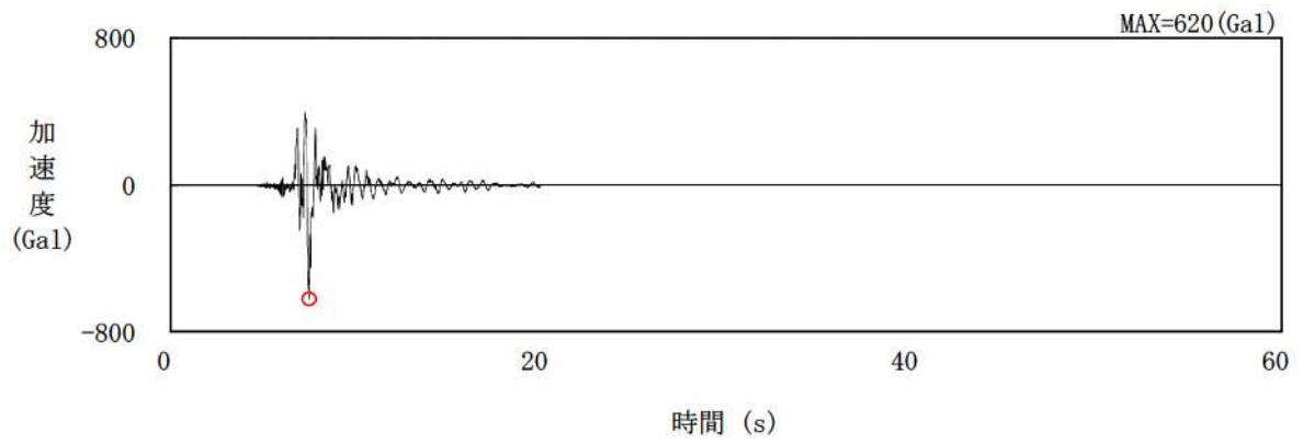
水平方向 : Ss3-4 (水平方向)
