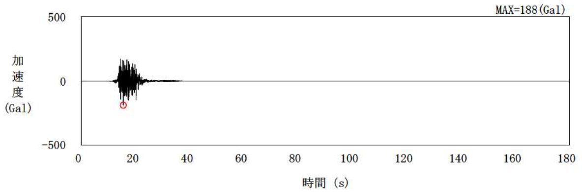
水平方向 : Sd2-11 (NS 方向)
