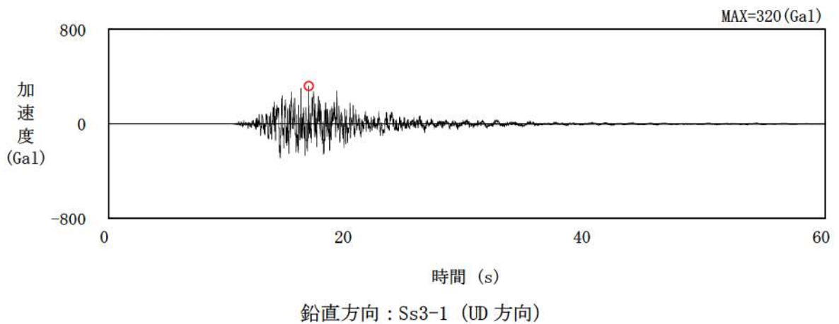
第5.17図 基準地震動Ss3-1の加速度時刻歴波形
