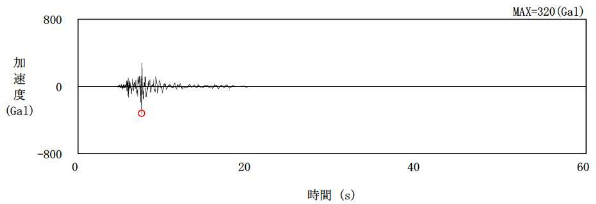
鉛直方向 : Ss3-4 (鉛直方向)
