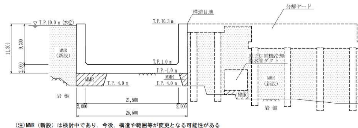
第5-59図 取水ピットポンプ室 断面図 (C-C 断面)
