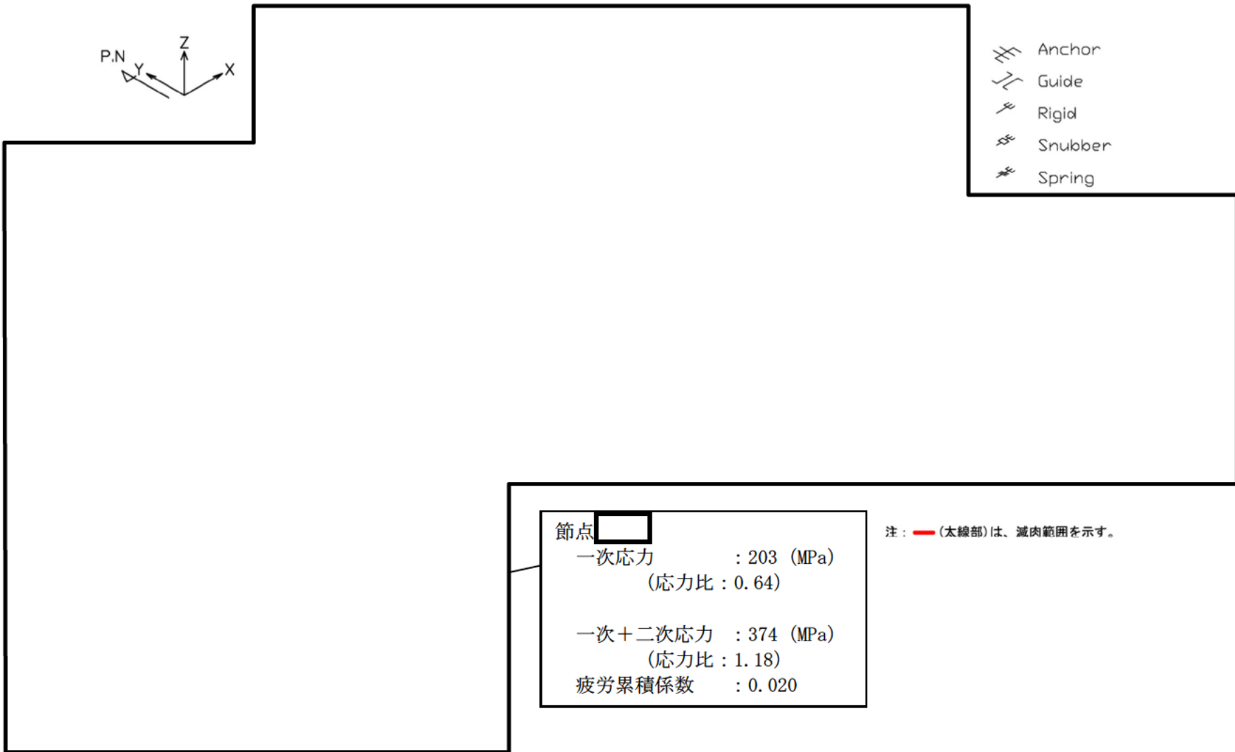
蒸気発生器ブローダウン系統配管 B-蒸気発生器ブローダウン配管 PEN#367CV外 CVBD内 【S s 地震】
