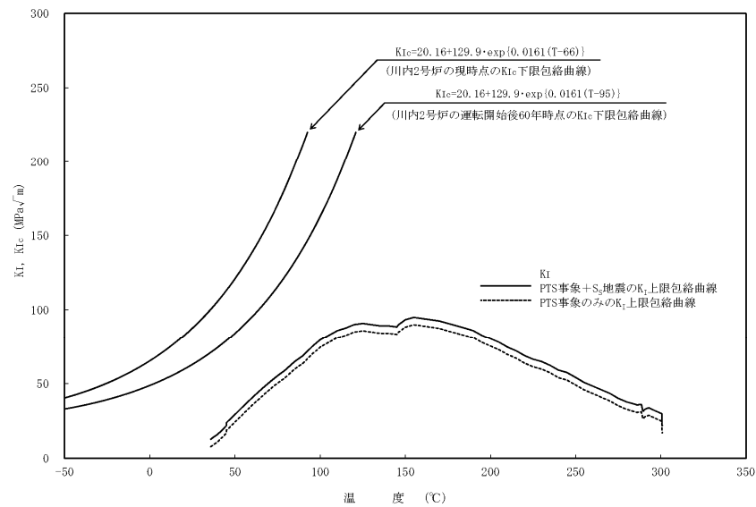
図 7-2 Ss 地震を考慮した PTS 評価結果
