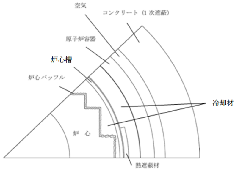
図 2-1 水平断面形状図 (R、 \theta 計算)
