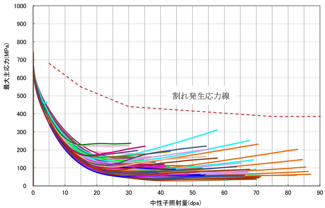
図 4-1 川内 2 号炉のバッフルフォーマボルトの応力履歴と割れ発生応力線の重ね合わせ (応力履歴は 50 万時間まで)
