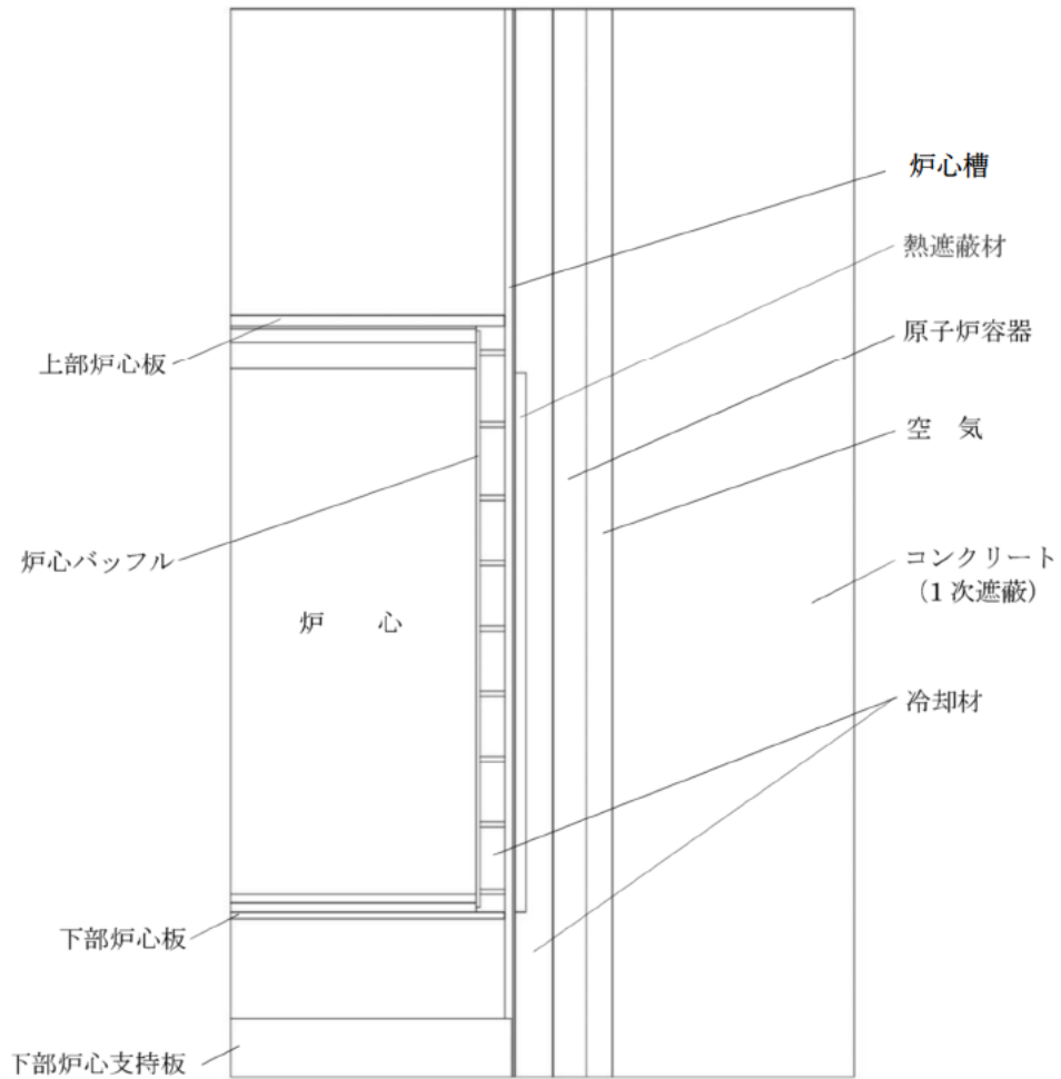
図 2-2 垂直断面形状図 (R、Z 計算)
