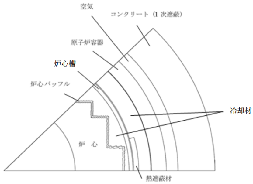
図 2-1 水平断面形状図 (R、 \theta 計算)
