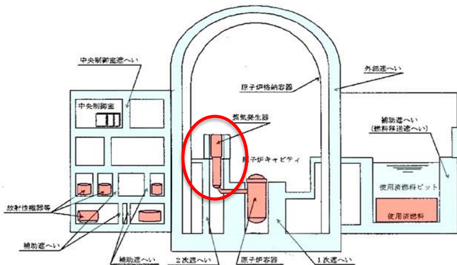
PWRの遮へい設備の構成
