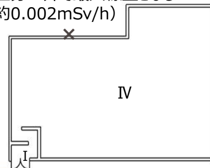
図 遮蔽設計区分概要図
