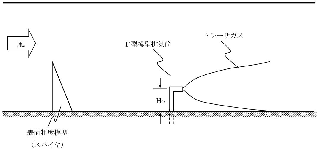
図 2.4-1 \Gamma 型模型排気筒によるトレーサガスの放出概念図
