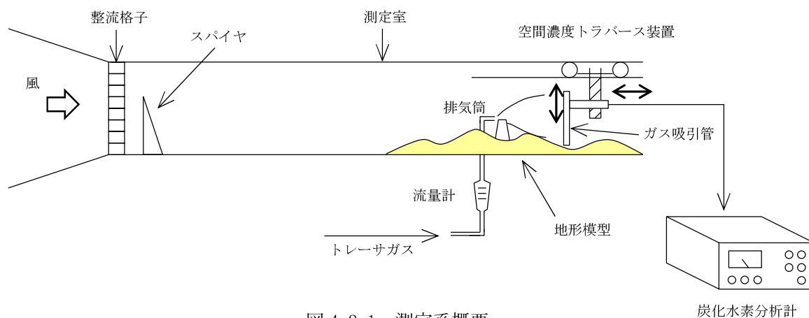
図 4.2-1 測定系概要
