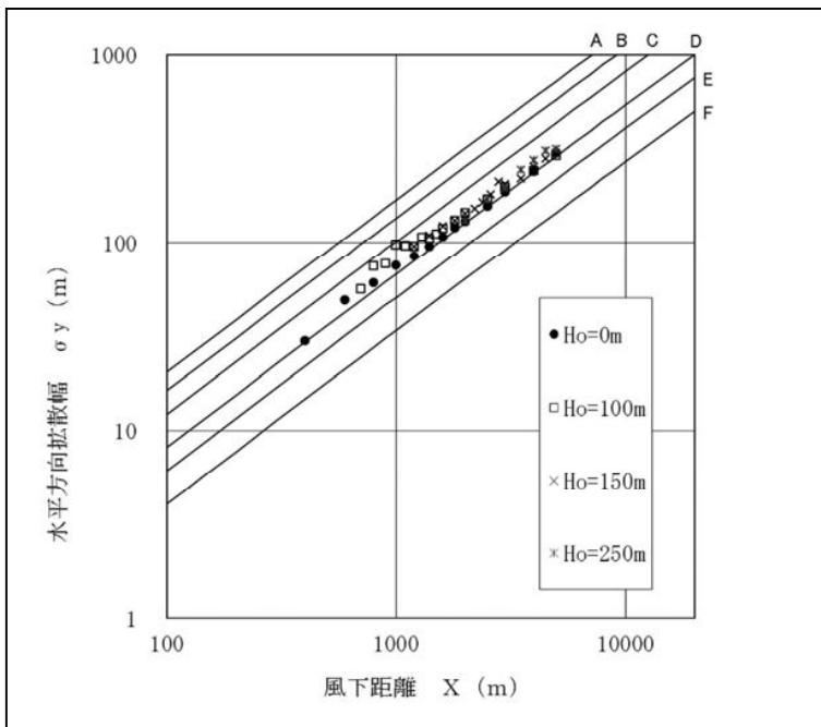
図2 風洞実験における大気水平方向の拡がり（気流条件）の新旧比較
