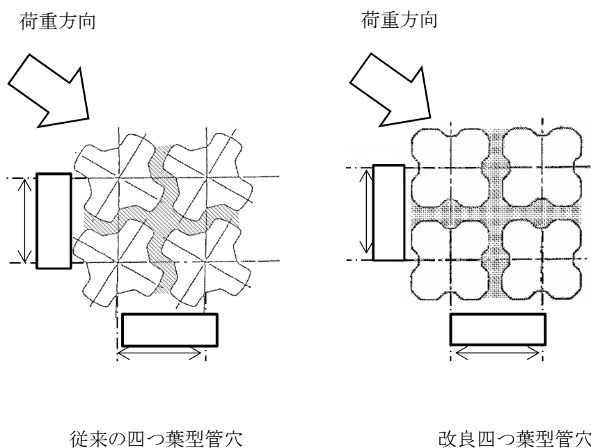
第 11-1 図 SG 取替え前後の管支持板管穴形状比較図
