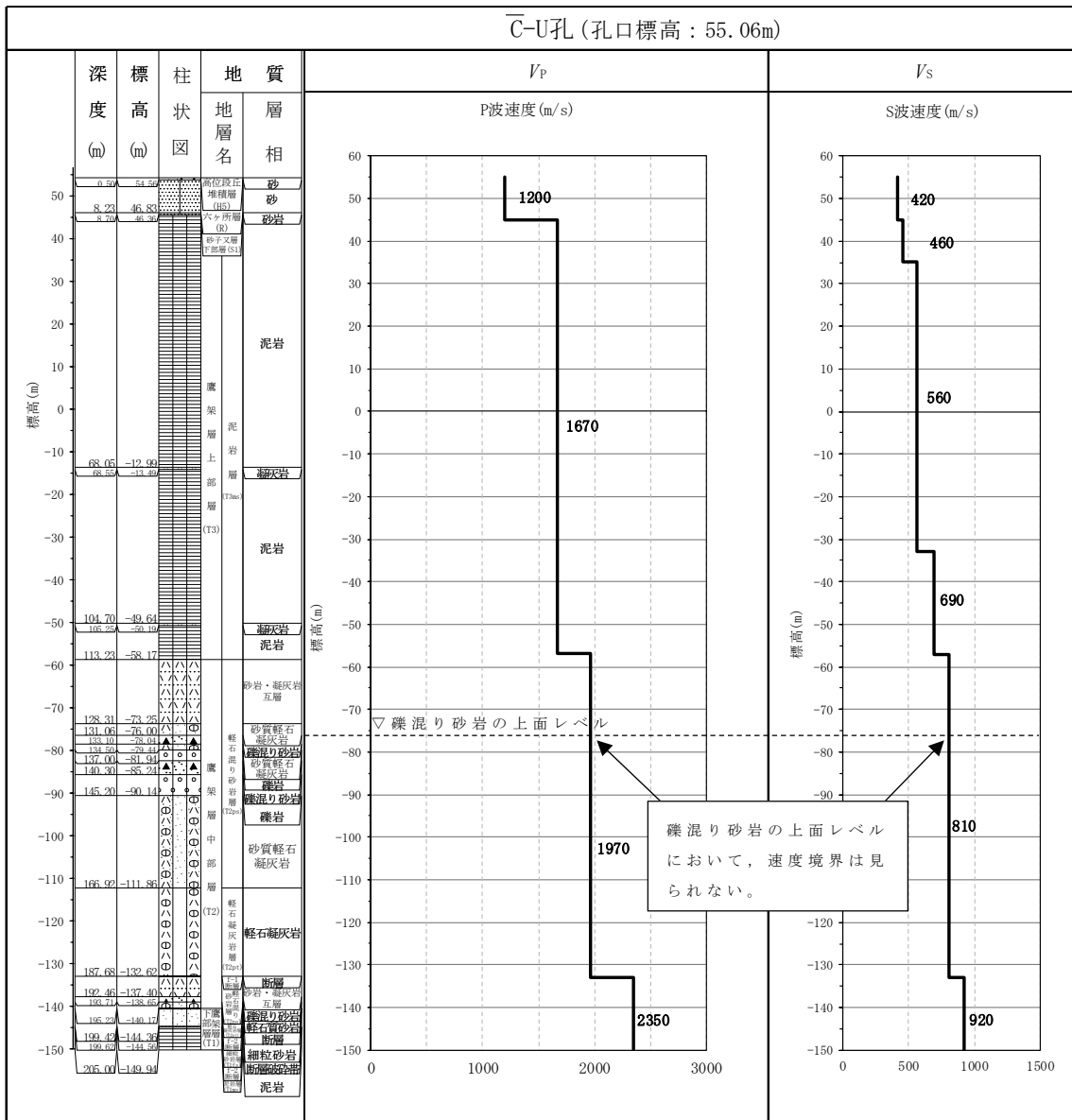
第 3.12-1 図 PS 検層結果 (E 施設周辺グループ) (4/5)
