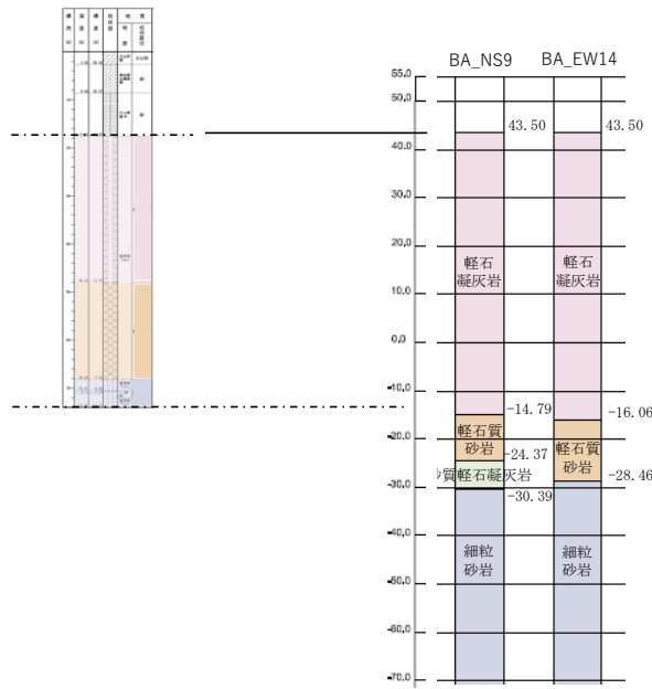
NS9とBA_EW14の 地下構造
