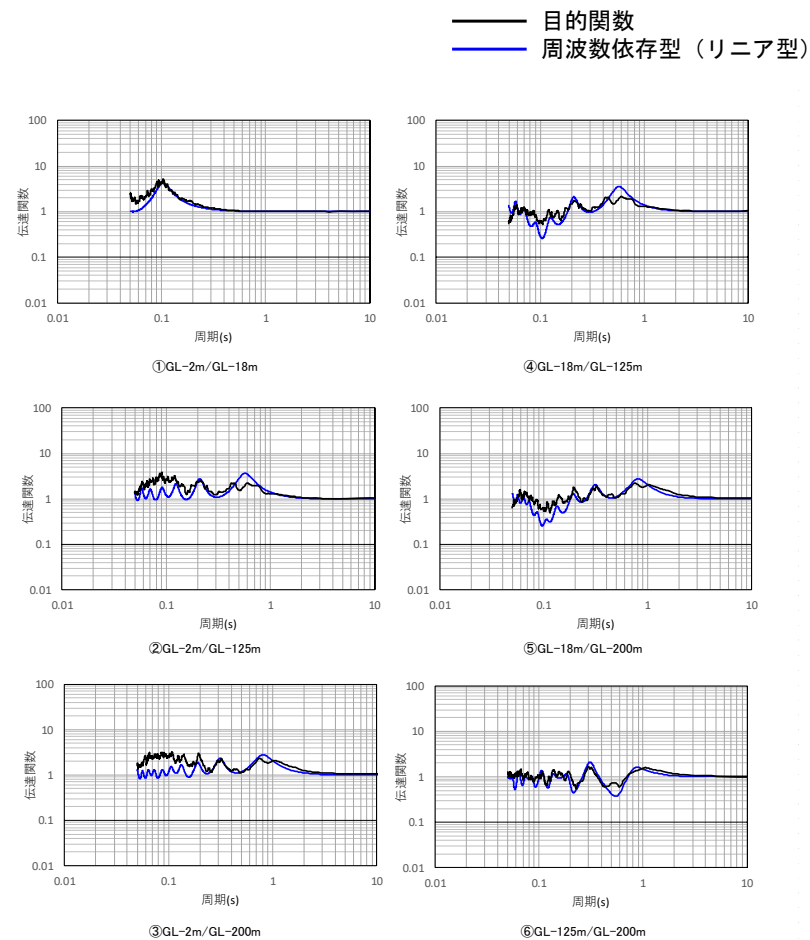
(b) 伝達関数適合状況
