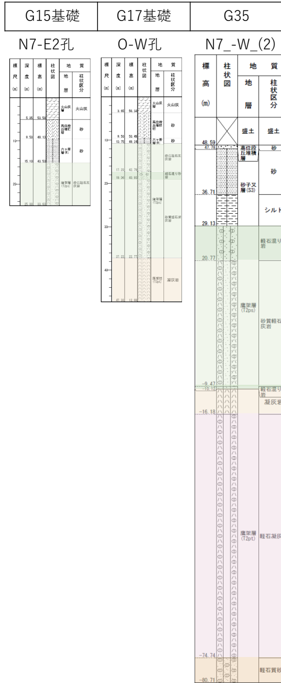
第 2-2 図 地質柱状図 (4/5)
