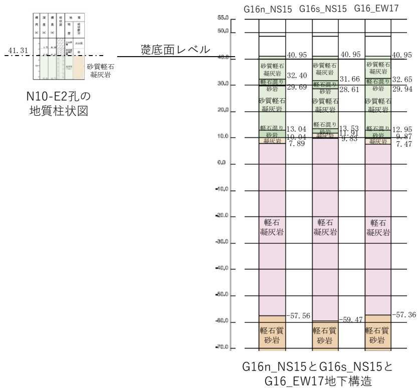
第3-20図 N10-E2孔及びG16直下の地下構造の対応
