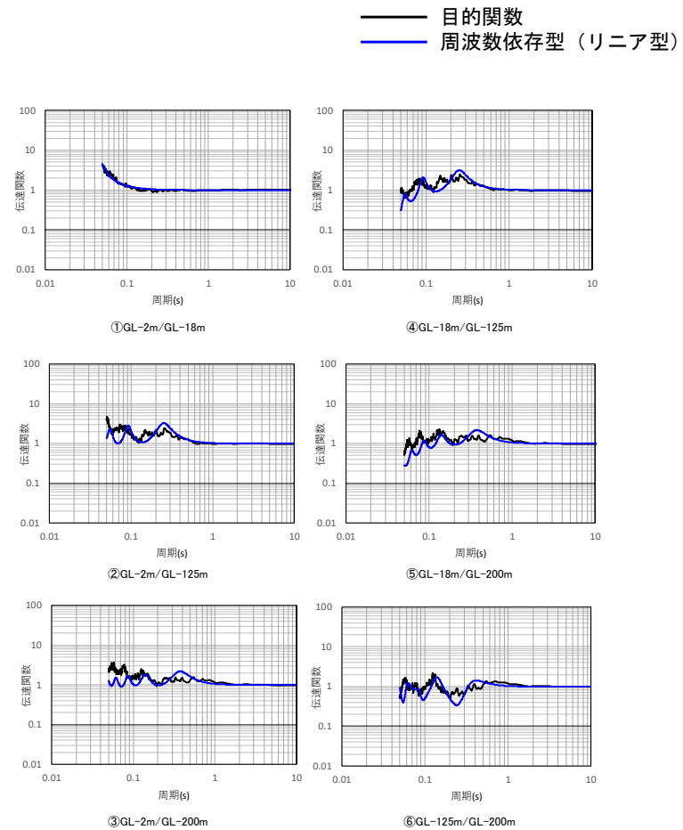
(b) 伝達関数適合状況
