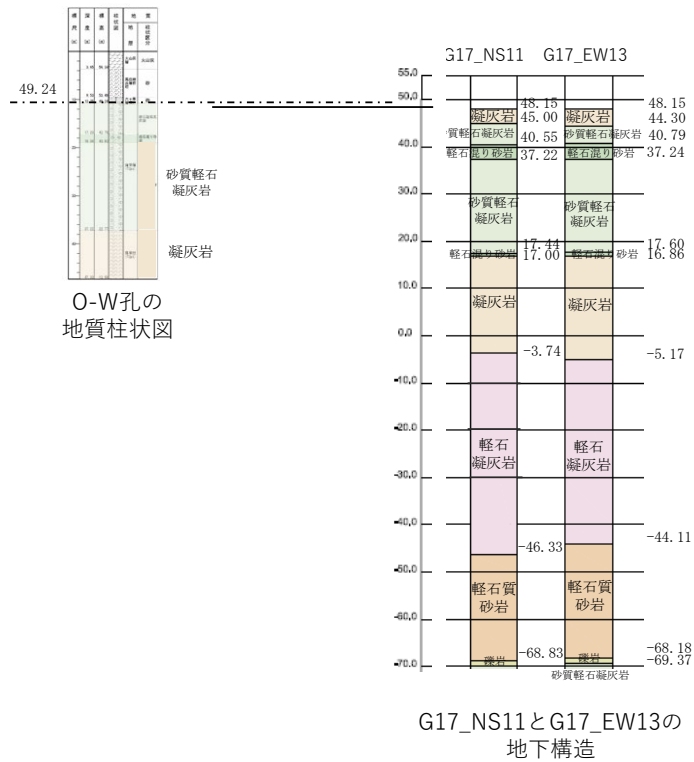
第3-19図 O-W孔及びG17直下の地下構造の対応
