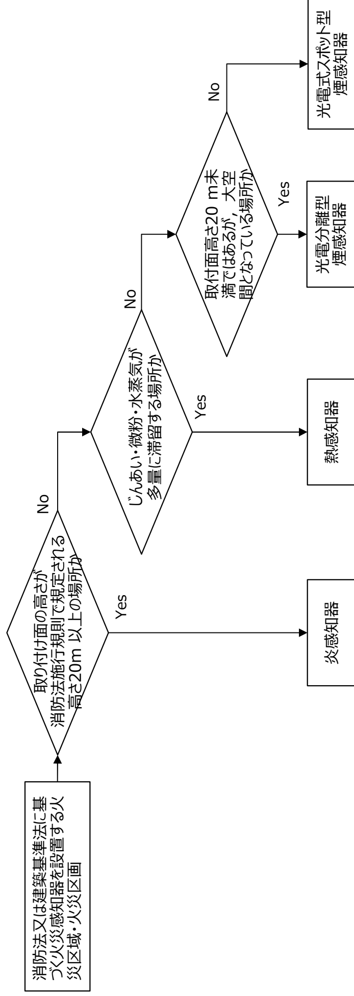
図5 火災感知器の選択フロー
