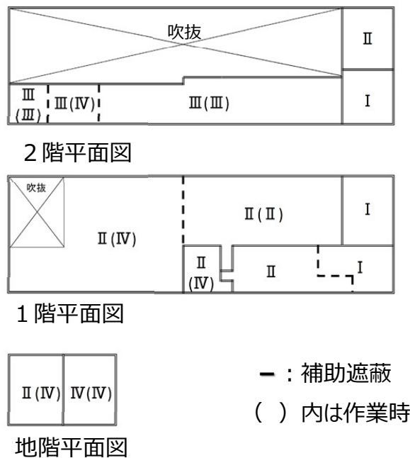
第6図 遮蔽設計区分概要図
