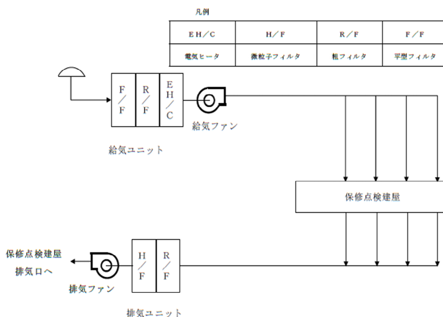
第7図 保守点検建屋換気系統概要図
