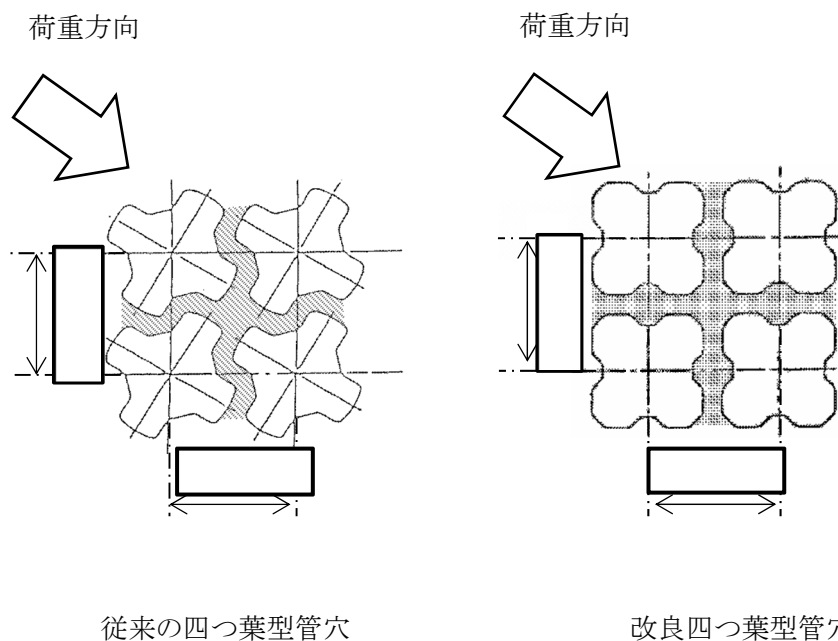
第 11-1 図 SG 取替え前後の管支持板管穴形状比較図
