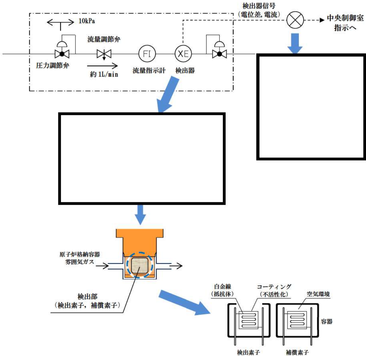
別図－3 可搬型格納容器内水素濃度計測ユニット（基本構造図）
