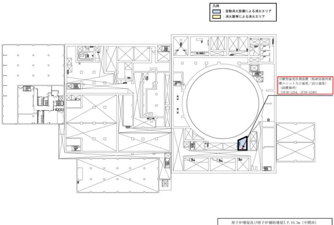
第 5 3 図 重大事故等発生時の計装設備の配置 (2 / 5)
