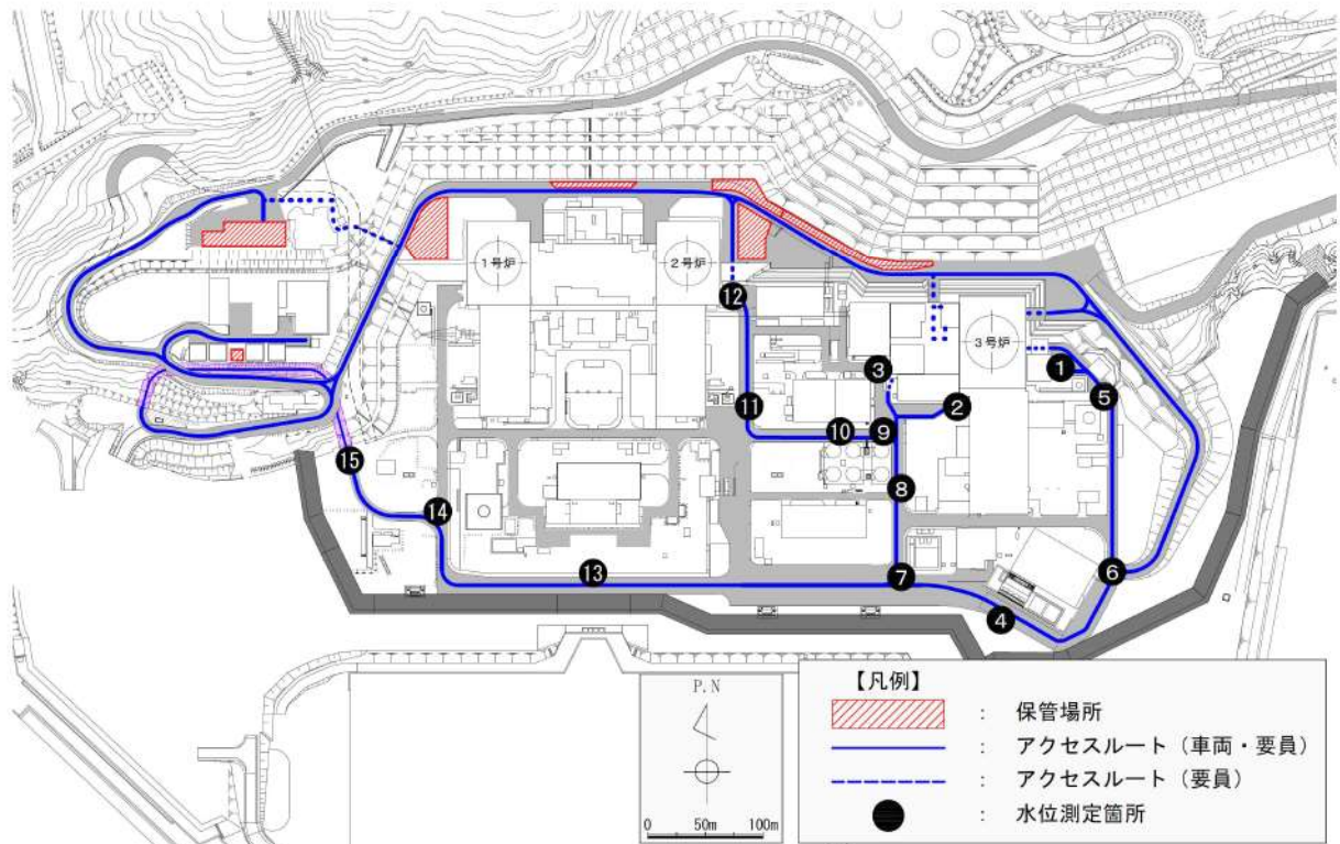
第5図 水位測定箇所
