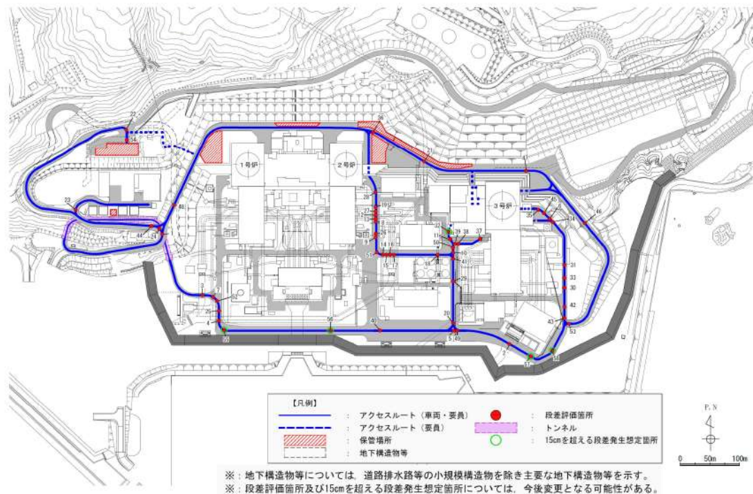
第5図 不等沈下による対策箇所
