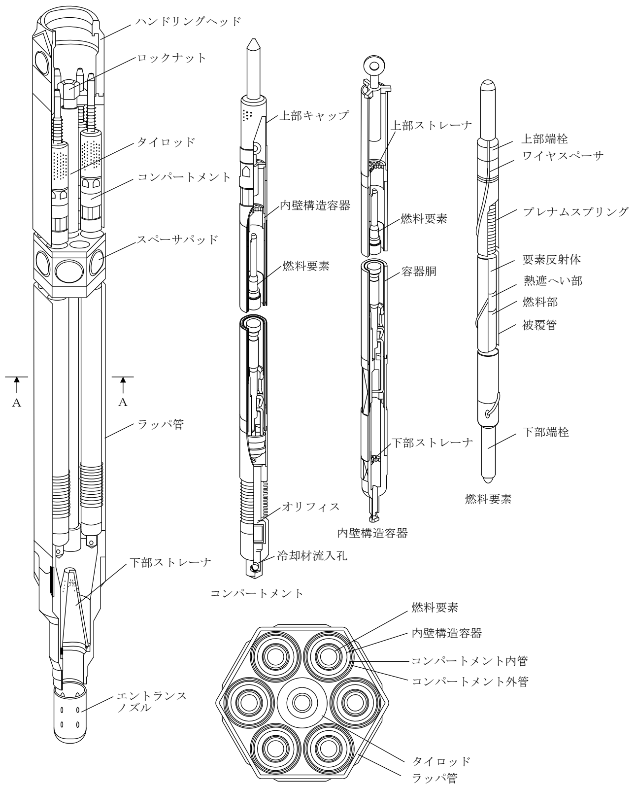
第3.7.7図 B型照射燃料集合体—先行試験用 (参考用)
