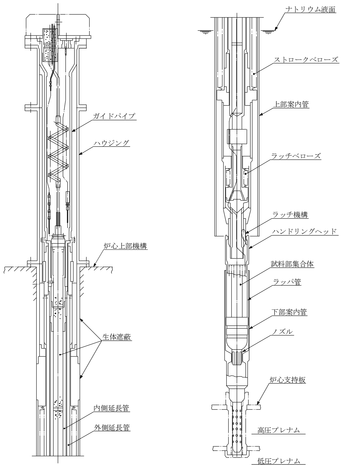
第 4. 1. 7 図 計測線付 C 型照射燃料集合体 (参考用)
