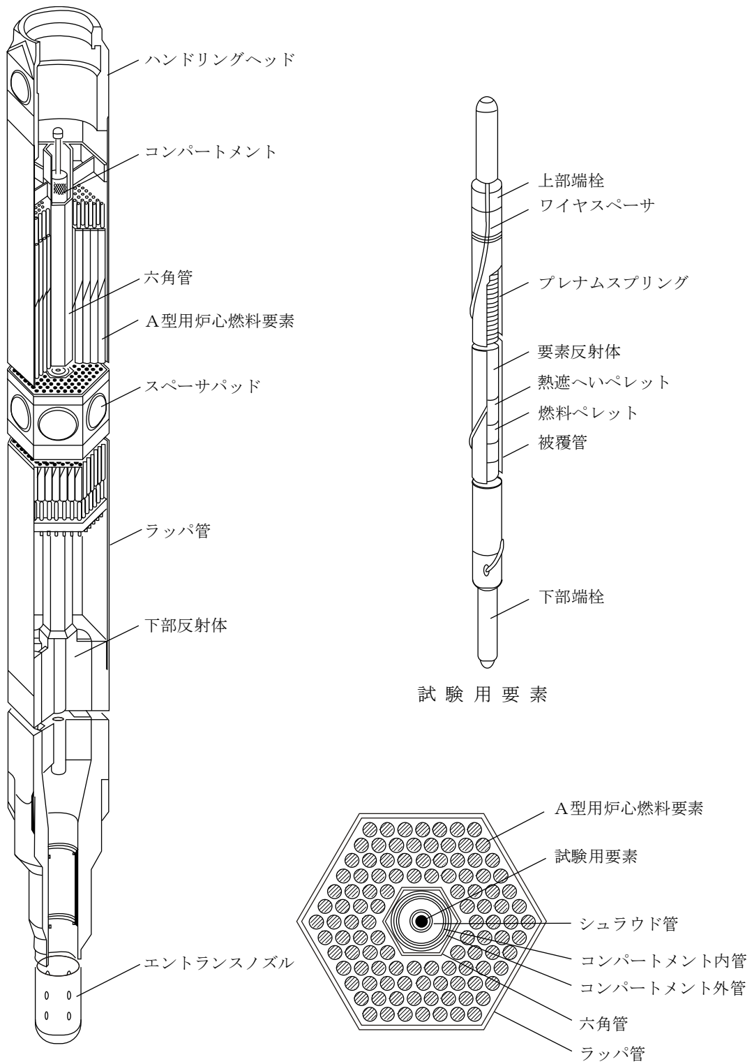
断面
