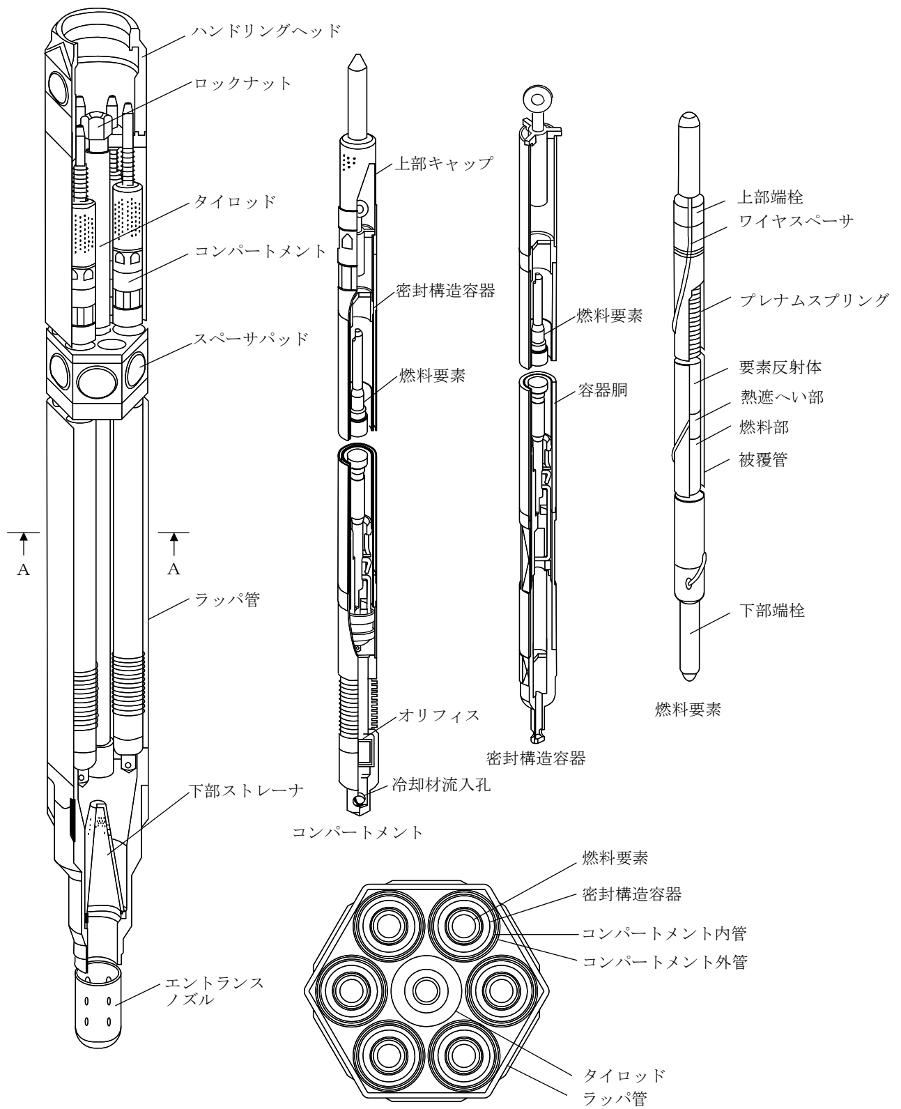
第3.7.8図 B型照射燃料集合体—基礎試験用 (参考用)
