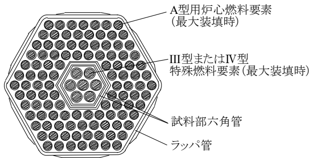
A型照射燃料集合体
