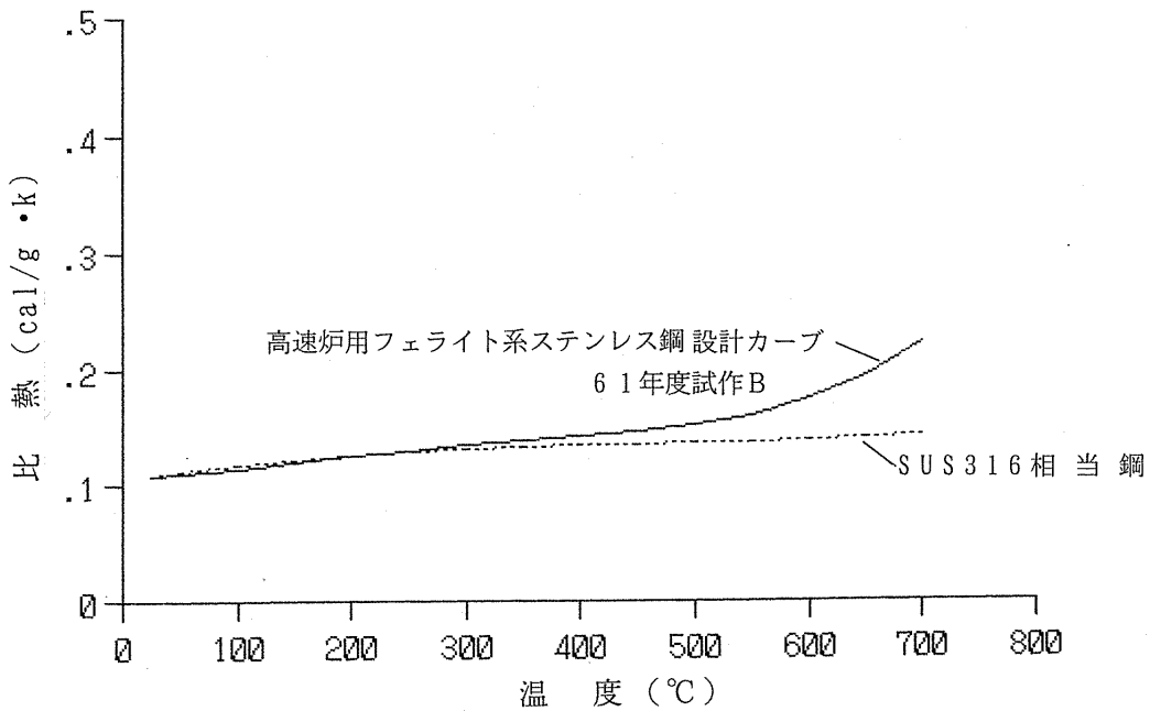
第 2.2.2 図 比熱
