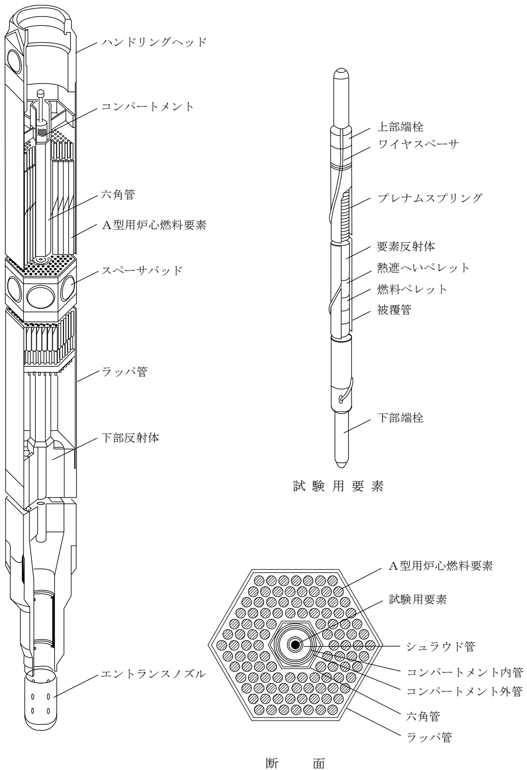
第 4.1.2 図 A型照射燃料集合体—限界照射試験用 (参考用)
