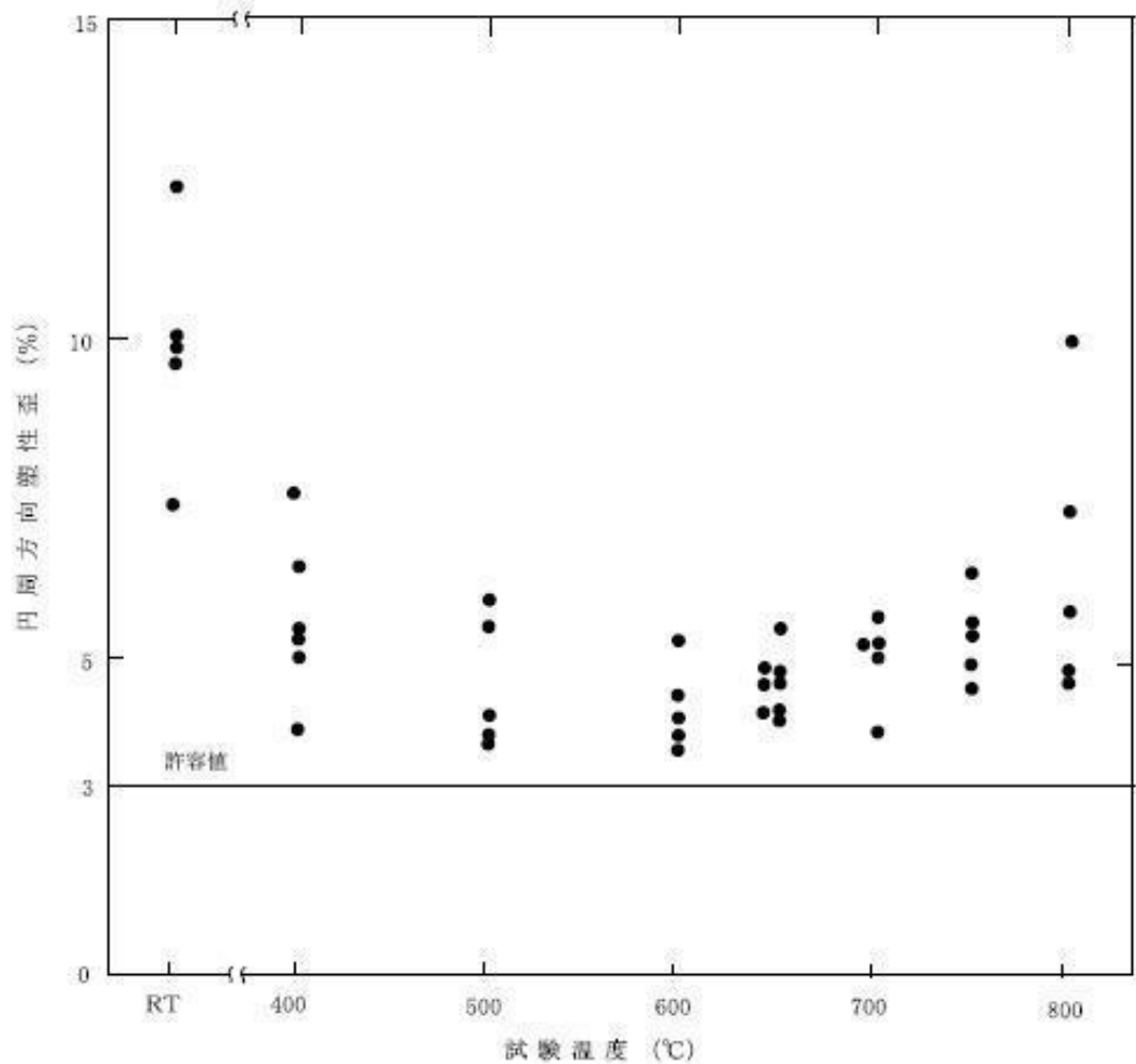
第2図 ステンレス鋼の破断歪
