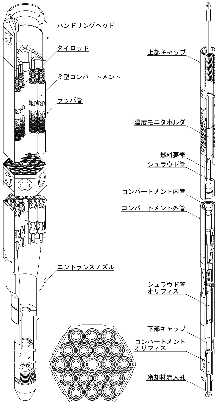
第 4.1.8 図 D型照射燃料集合体－ \delta 型コンパートメント最大装填型 (参考用)
