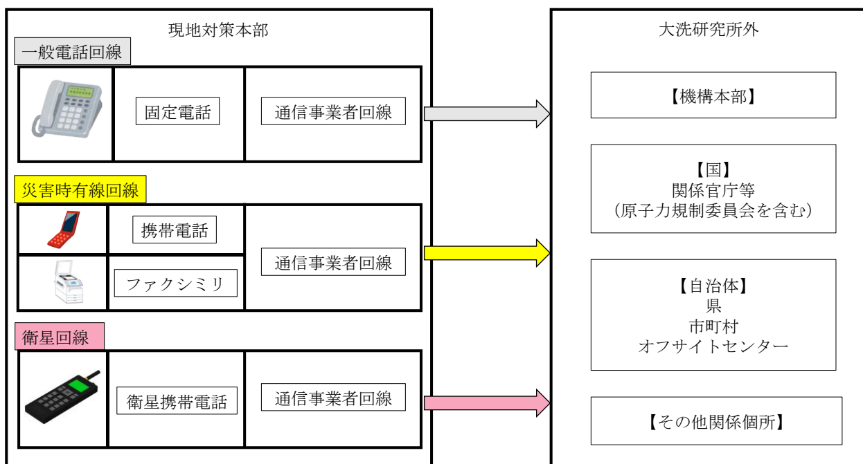
第 1 図 外部通信連絡設備と外部必要箇所
