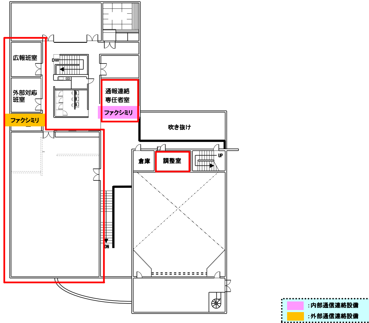
緊急時対策所における通信連絡設備の配置図 (1/2)
