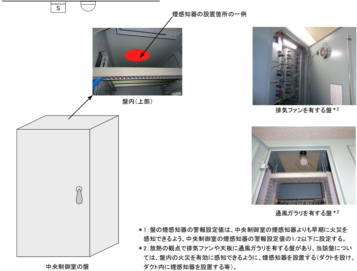
第 2.1 図 中央制御室の盤に対する煙感知器の設置イメージ
