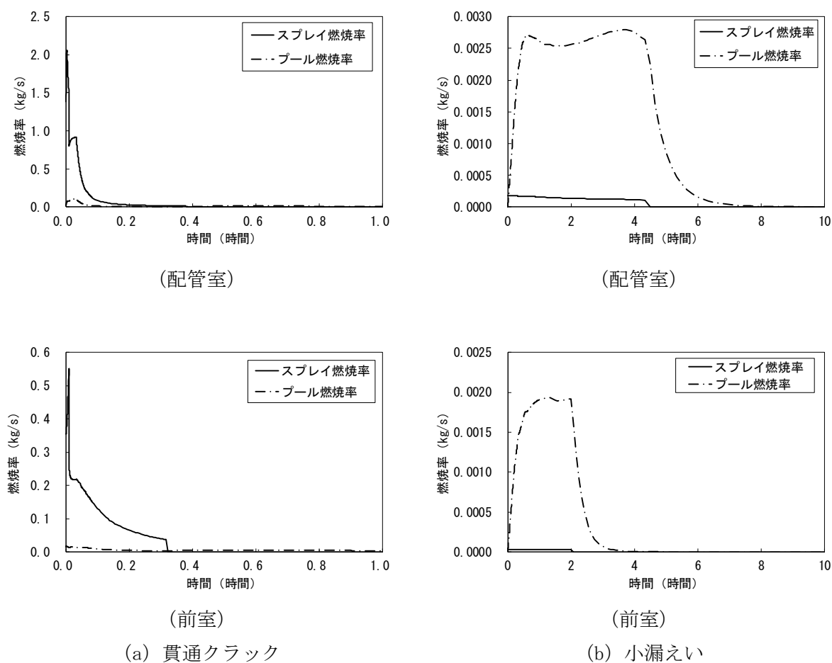
第 1 図 スプレイ及びプール燃焼率の時刻歴変化
