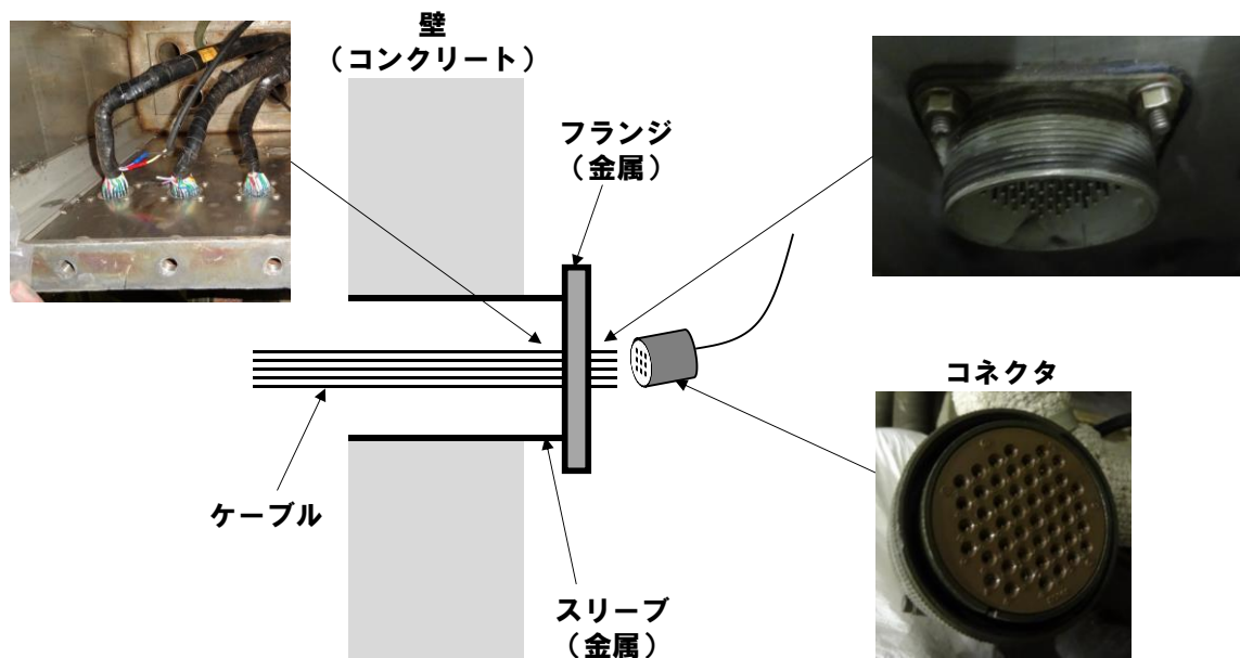
第 3.1 図 ケーブルの配線の概略図
