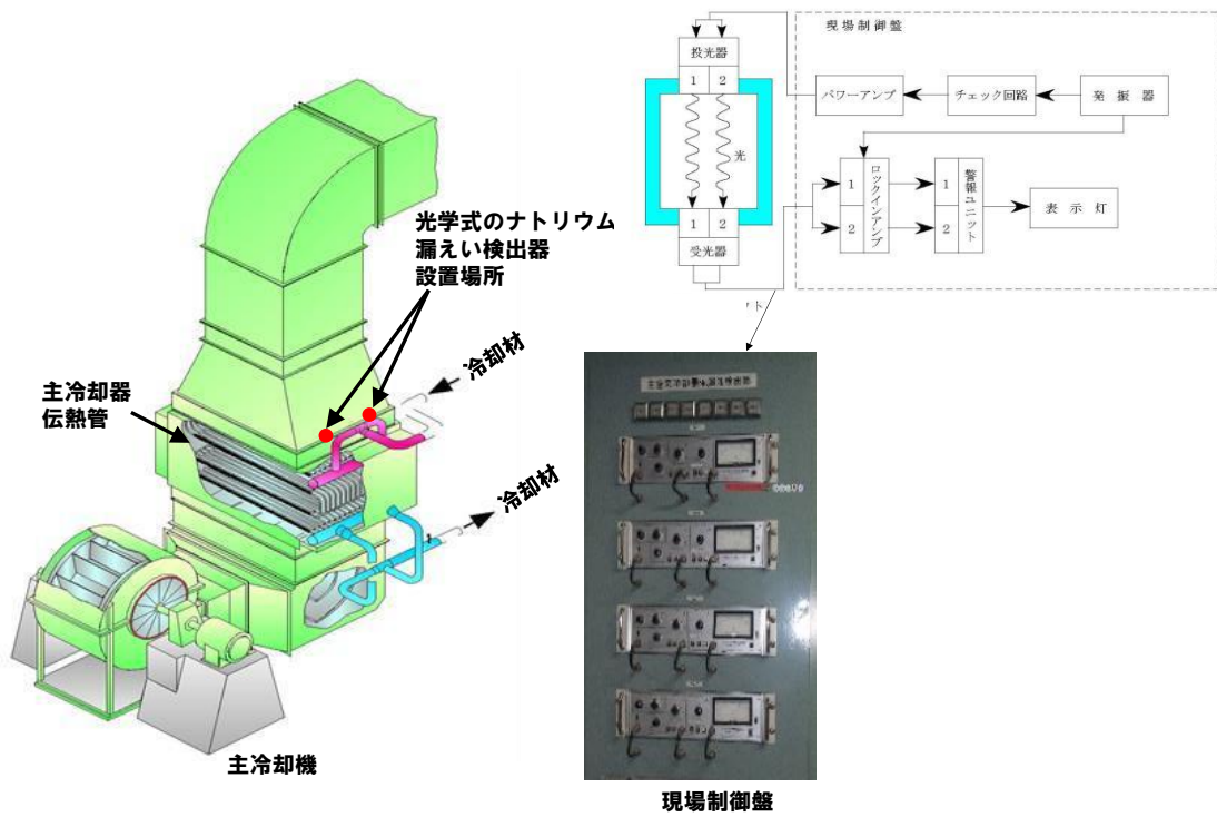
第 2.1.4 図 光学式のナトリウム漏えい検出器の構造概要
