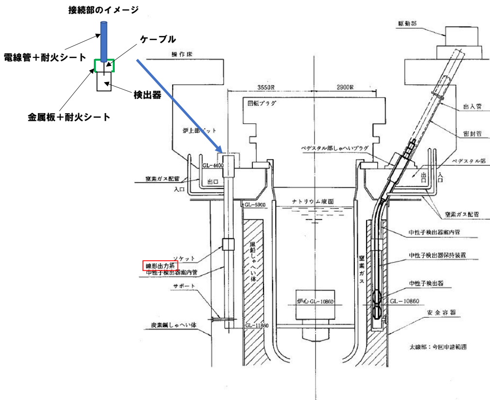
(断面図)
