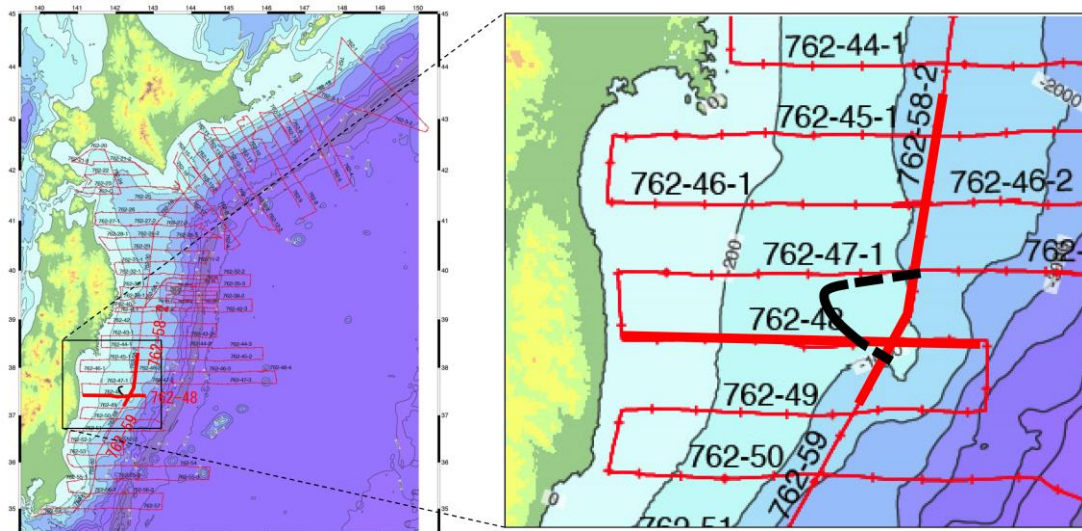
測線図
