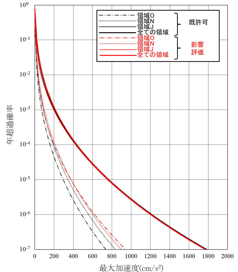
図4 領域ごとのハザード曲線の比較 (萩原マップ)
