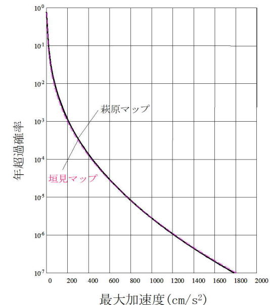
図3 萩原マップ及び垣見マップのハザード曲線の比較 (既許可時)
