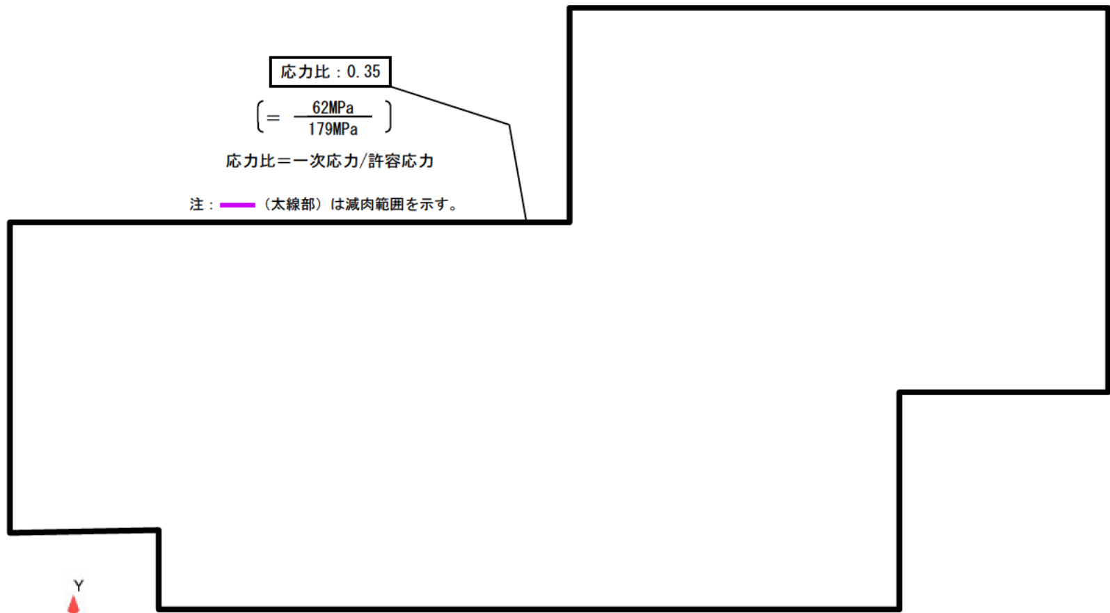
補助蒸気系統配管 スチームコンバータ発生蒸気管
