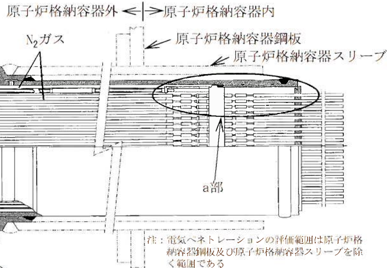
構造図
