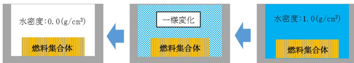
第1-1図 既工事計画における未臨界性評価体系
