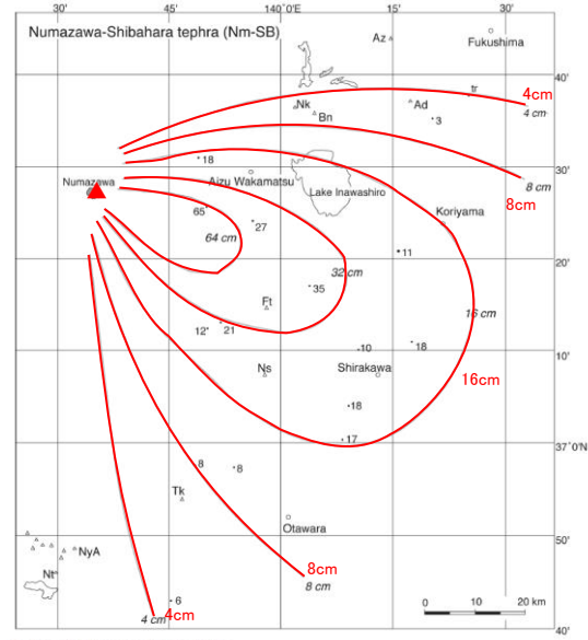
第38図 沼沢芝原テフラ (Nm-SB) の分布。 数字は降下火砕堆積物の層厚で、単位は cm。Ad = 安達太良火山; Az = 吾妻火山; Bn = 磐梯火山; Ft = 二岐山火山; Nt = 男体火山; Nm = 沼沢火山群; Nt = 男体火山; NyA = 女峰赤塚火山; Tk = 高原火山。山元 (2003) を一部改変。
