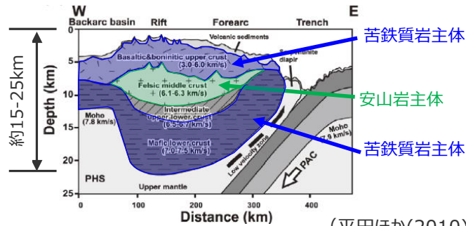
伊豆小笠原弧の地殻の模式図 (平田ほか(2010)を基に作成)
