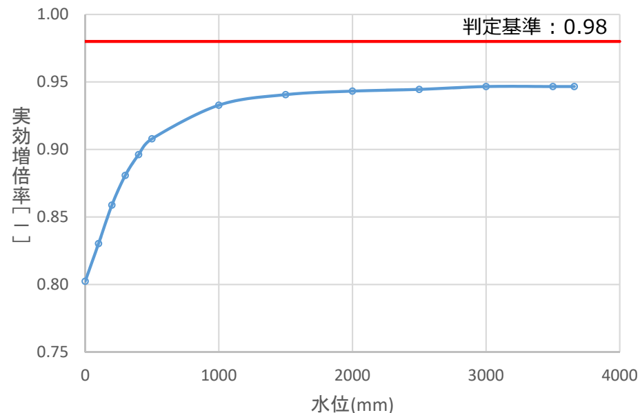
図1-2 実効増倍率評価結果
