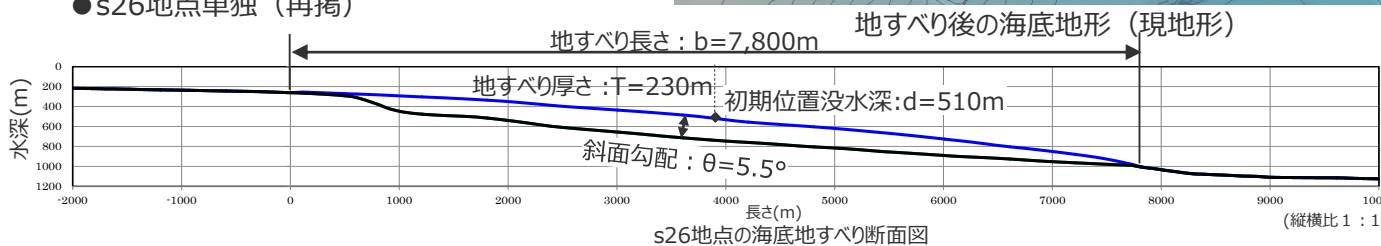
s26地点の海底地すべり断面図
