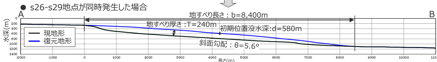
s26-s29地点が同時発生した場合の海底地すべり断面図
