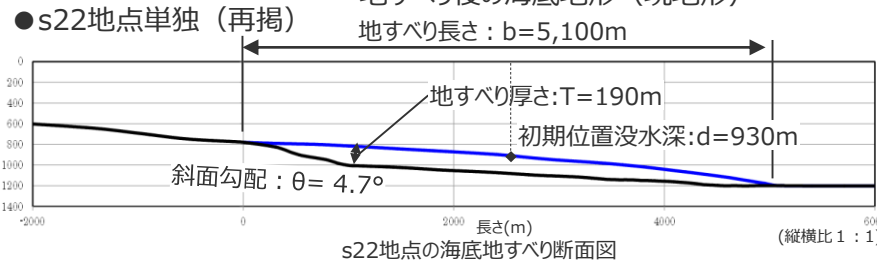
地すべり後の海底地形 (現地地形)
