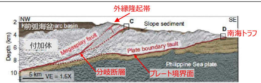
＜南海トラフを切る反射断面（左図B断面）＞ (地震調査委員会(2013)に図の説明（南海トラフ、プレート境界面、外縁隆起帯、分岐断層、前弧海盆、付加体）を加筆)
