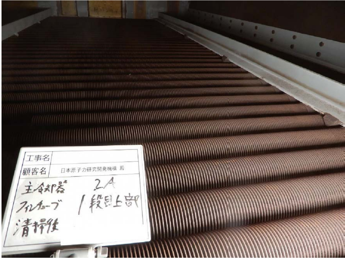
主冷却器伝熱管外観（令和5年1月時点）
