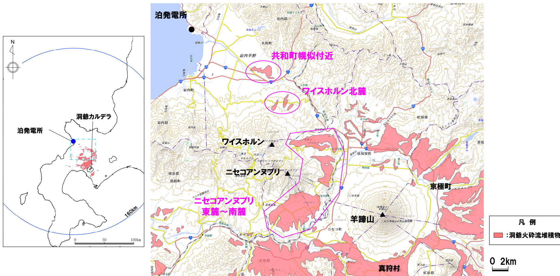
洞爺火砕流堆積物の分布範囲 (産業技術総合研究所地質調査総合センター編(2020)に加筆)
