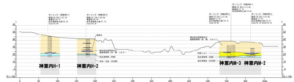
1-1'断面
