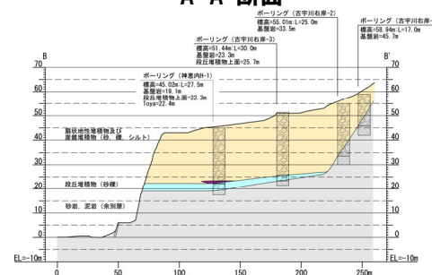
B-B'断面
